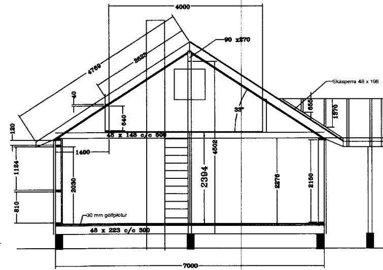
SNÍÐ A-A
