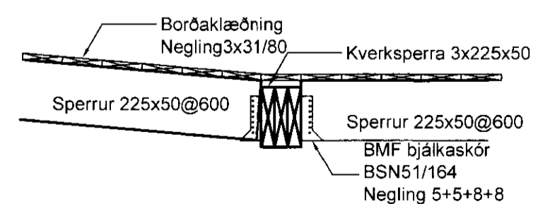
4 Snið þak 1:20
