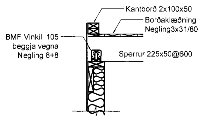
2 Snið þak 1:20
