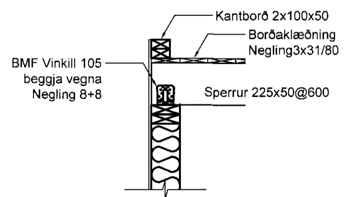
3 Snið þak 1:20
