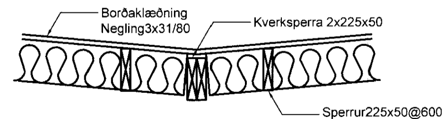
5 Snið þak 1:20
