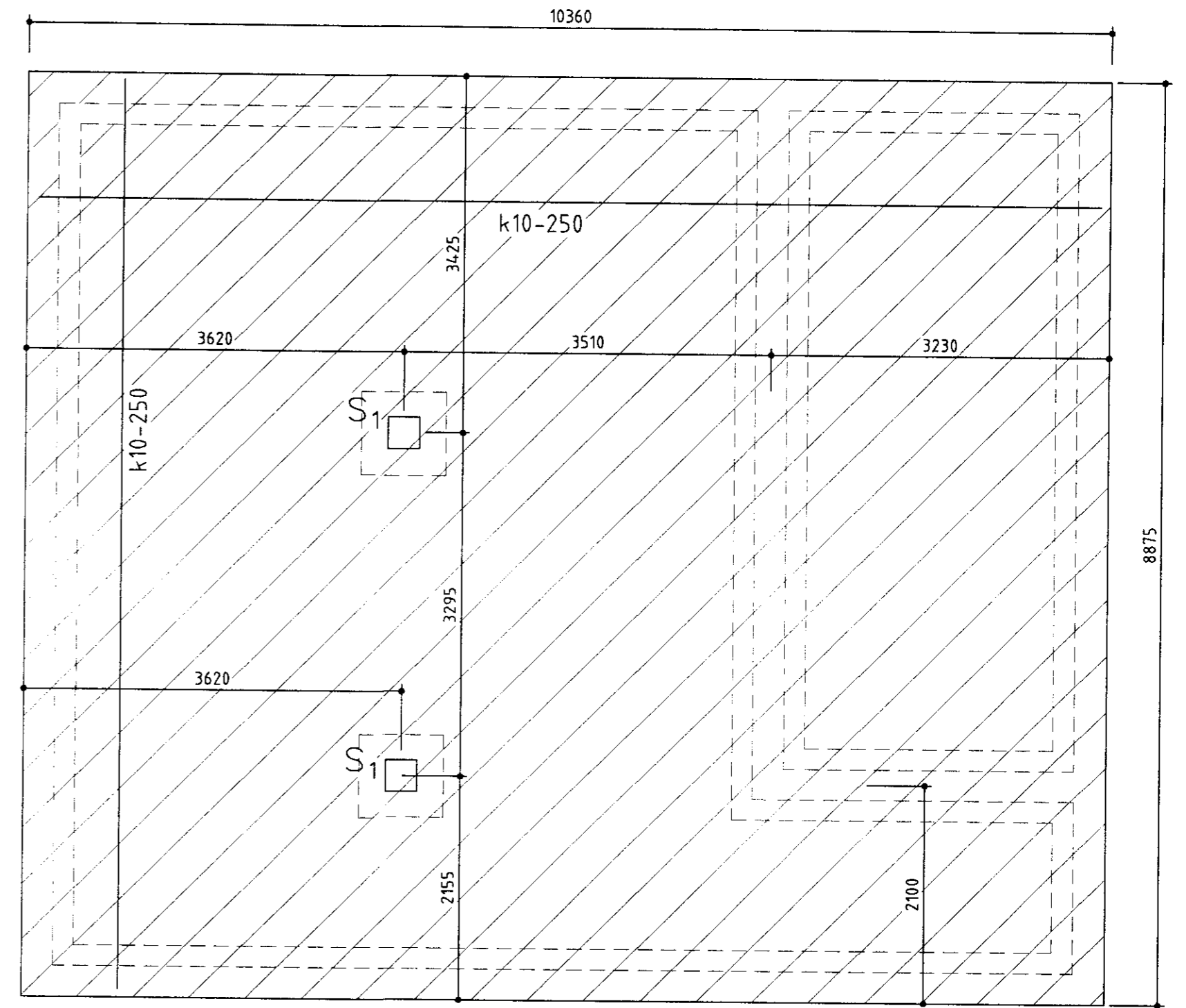
Kjallaraplata Mkv. 1:50
