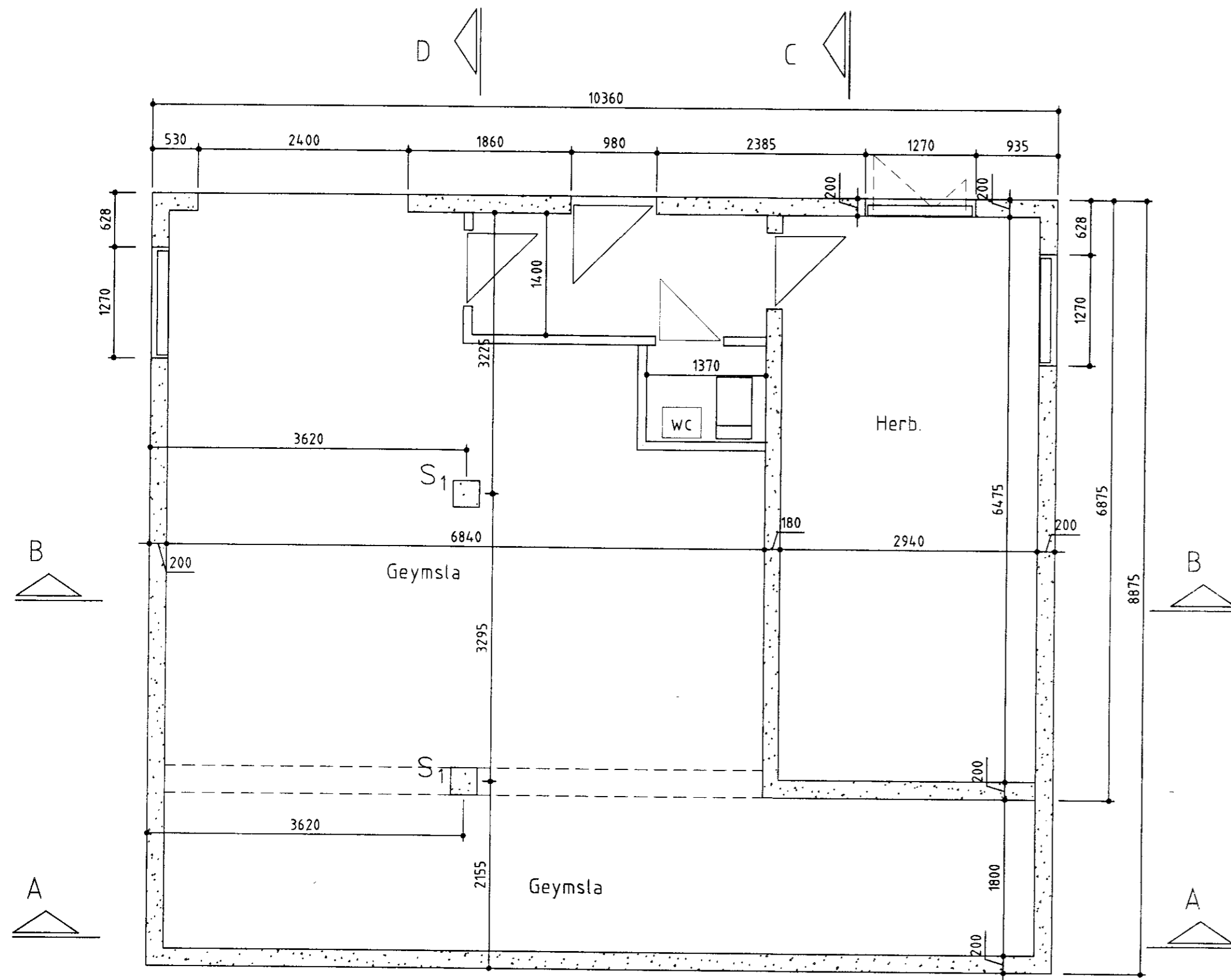
Kjallari Mkv. 1:50
