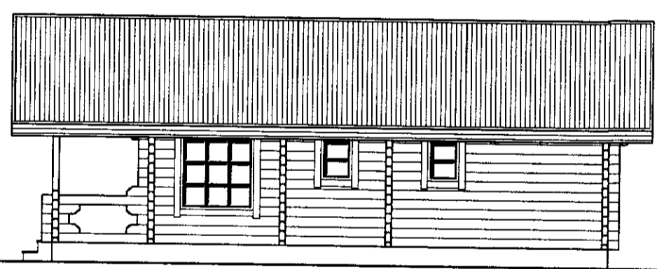
ÚTLIT NORDVESTURHLID
