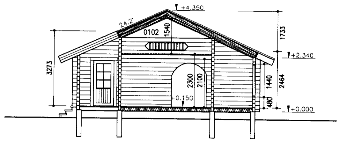
SNID A-A 1:100
