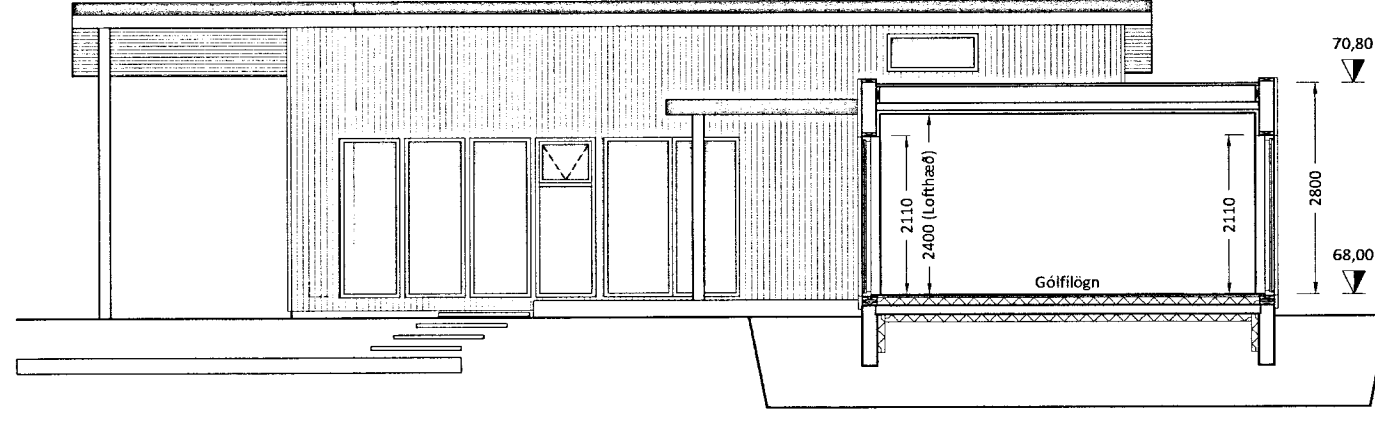
SNID B-B Mkv. 1:100
