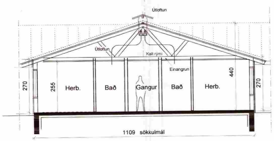
SNID B - B mkv. 1 : 100
