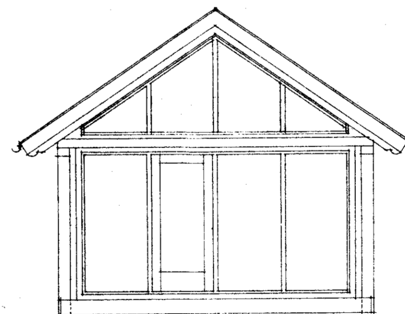
SÚÐLAGUR GAFL
