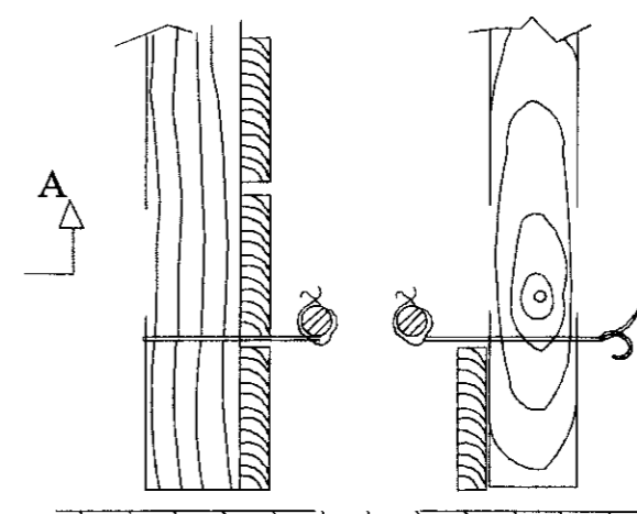
Snið A - A í sökkulvegg
