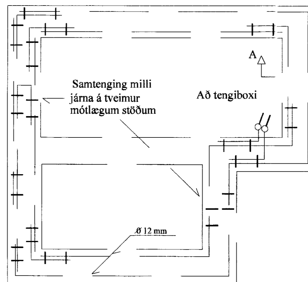
GRUNNMYND SÖKKULVEGGJA
