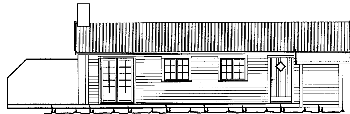
HLID NR. 2. 1:100
