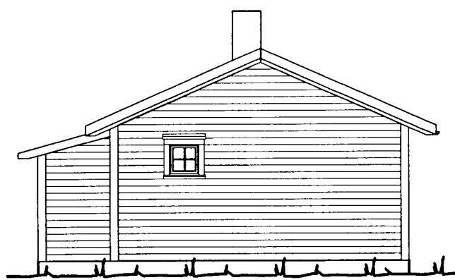
VEGGUR NR. 3. 1:100
