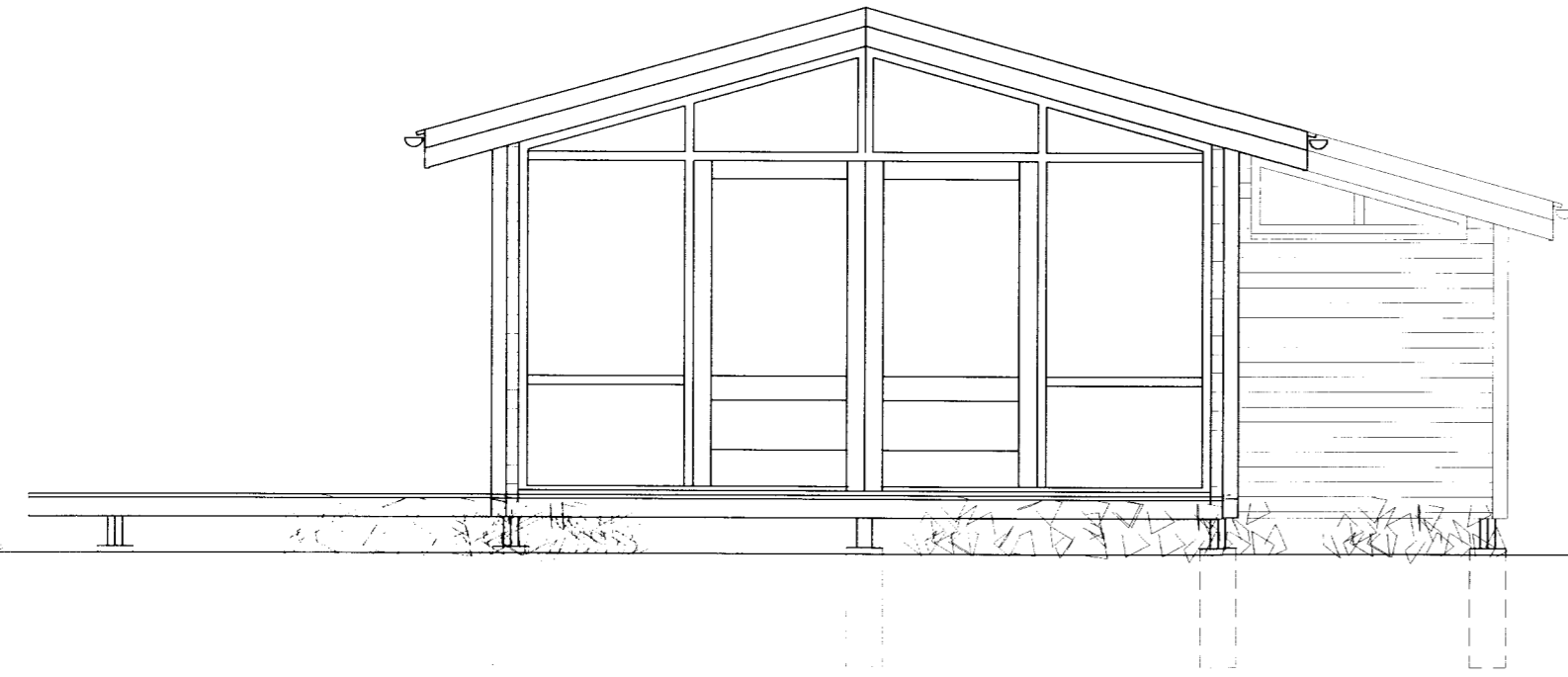
SUÐURGAFL
