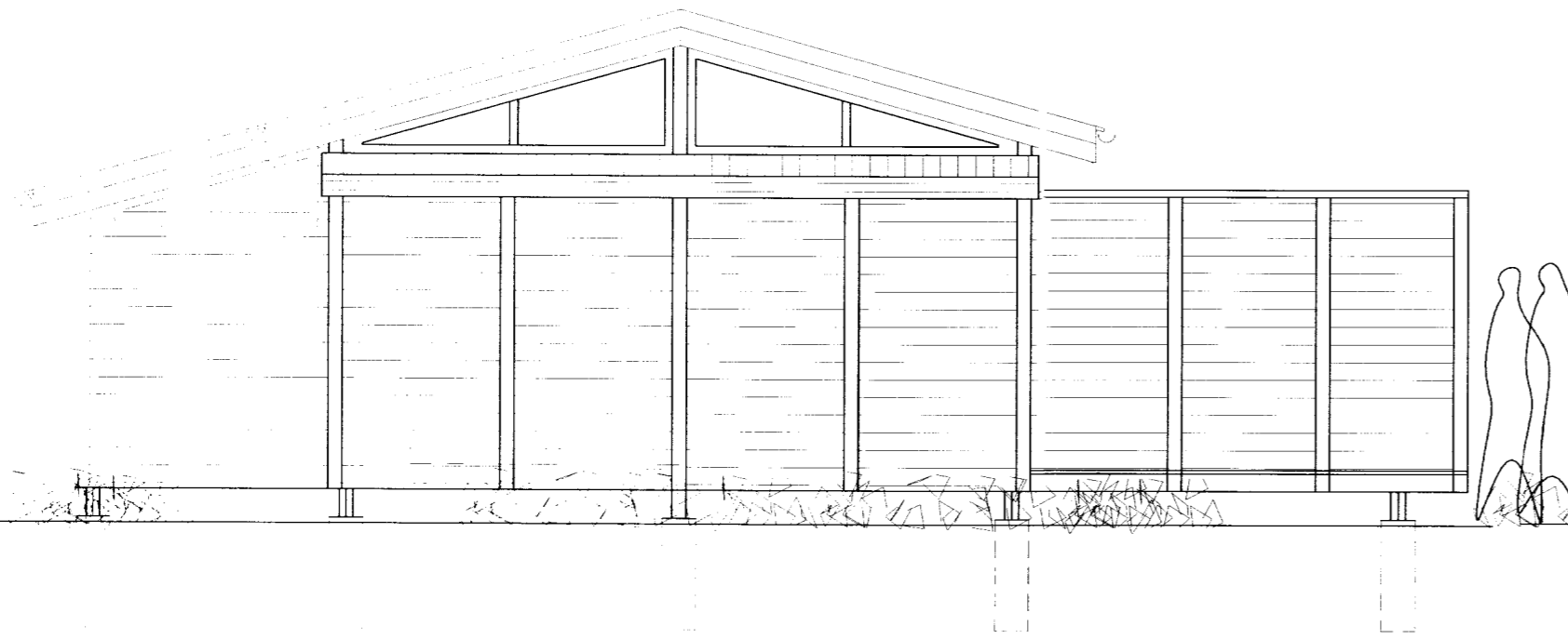
NORÐURGAFL
