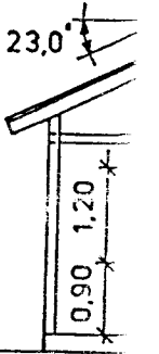
Snið
