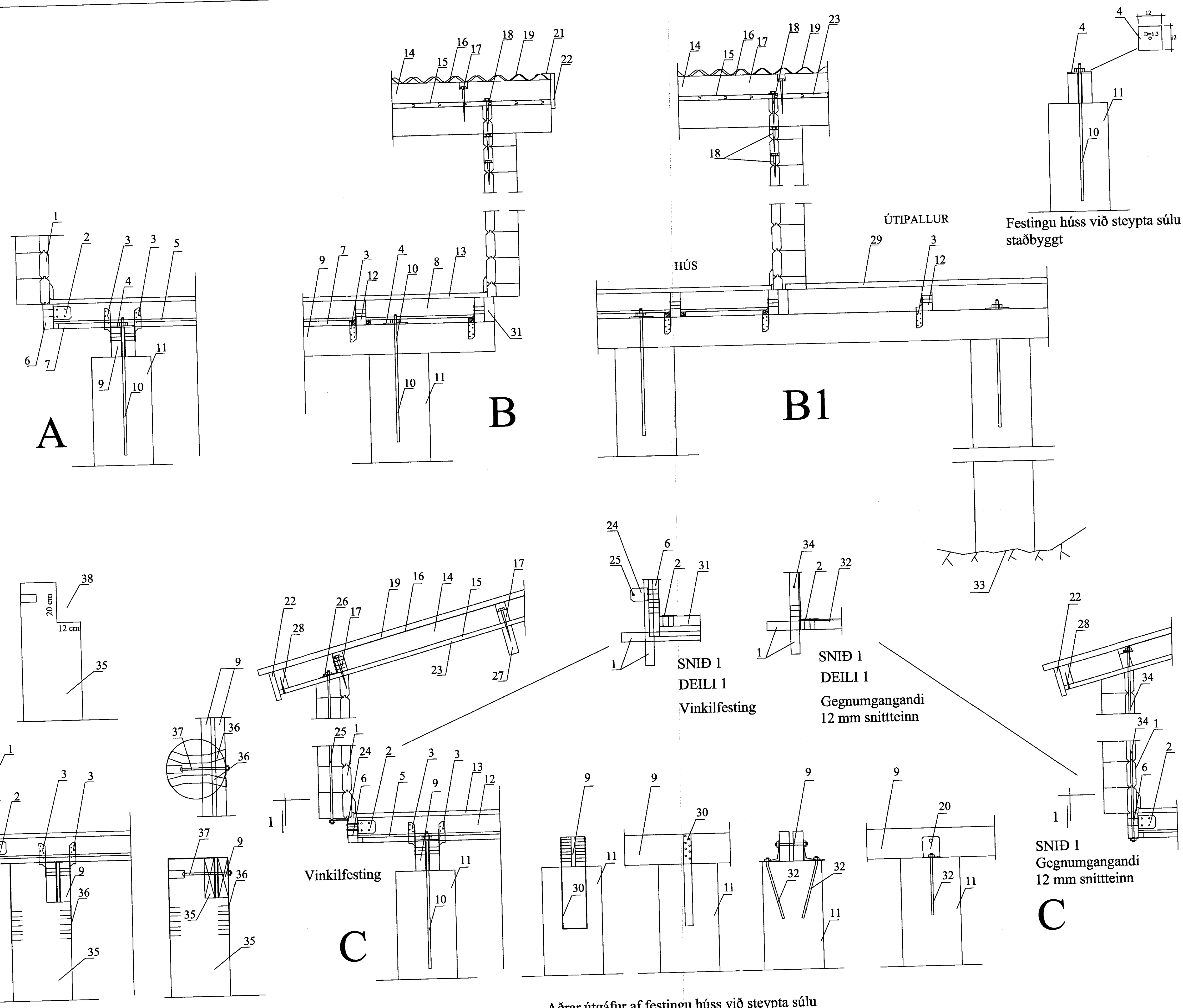
FESTING DREGARA VIÐ STAURA SÚLU
