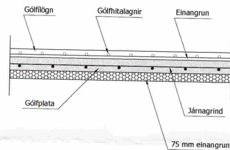
Snið í hitalagnir íbúðarýmis Mkv: 1:20
