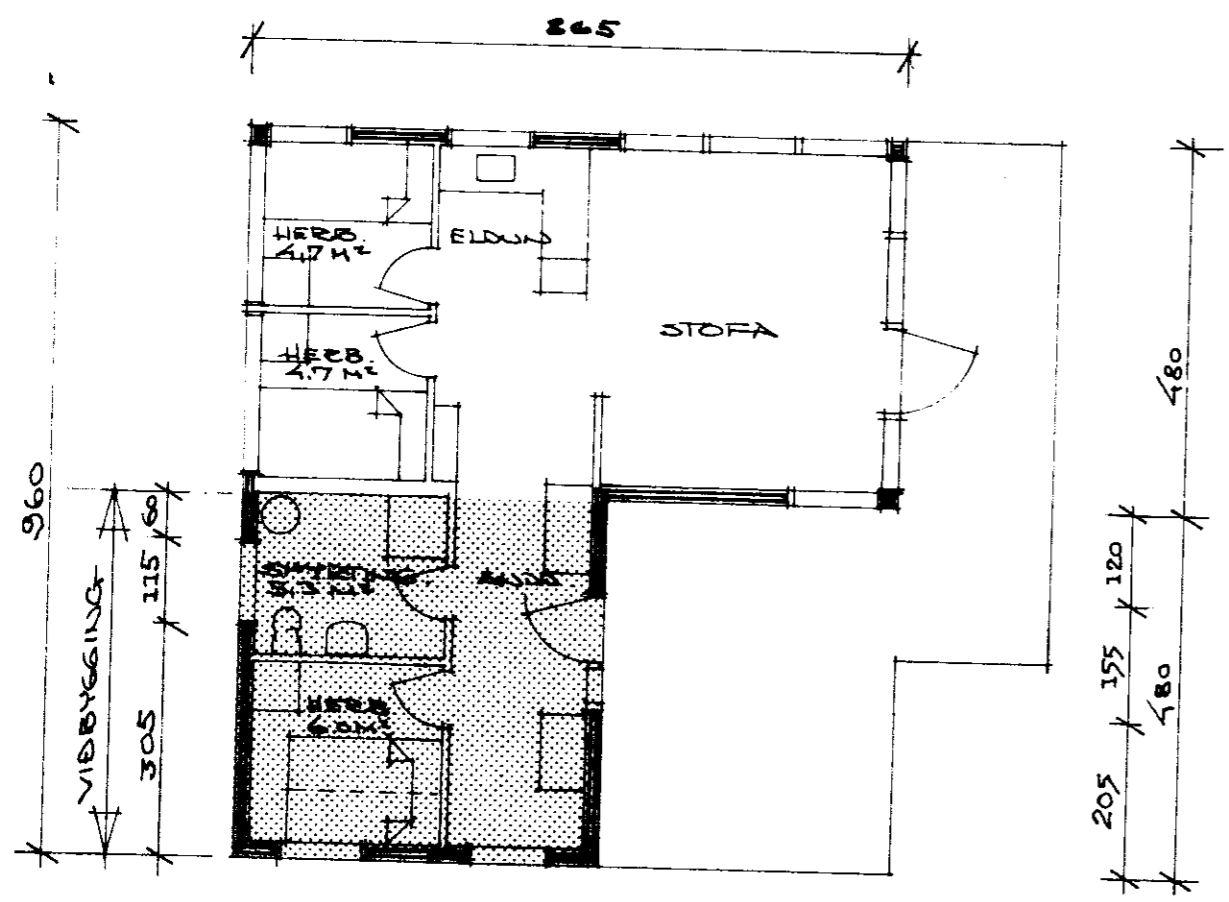
GRUNNMYND 1:100
