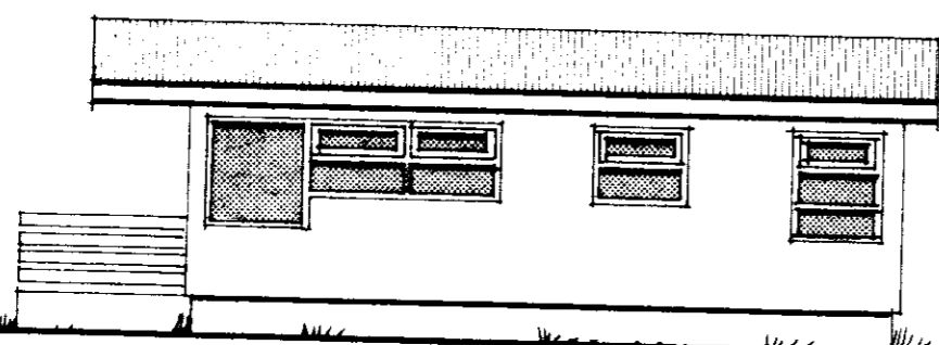
AUSTUR 1:100
