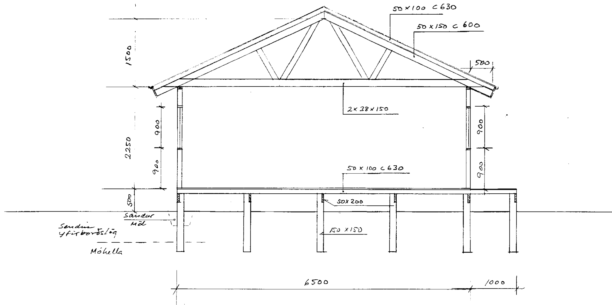
ÞVERSNIÐ 1:50
