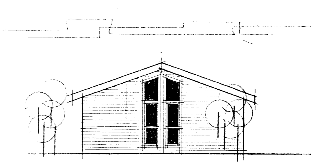
norð-austur
