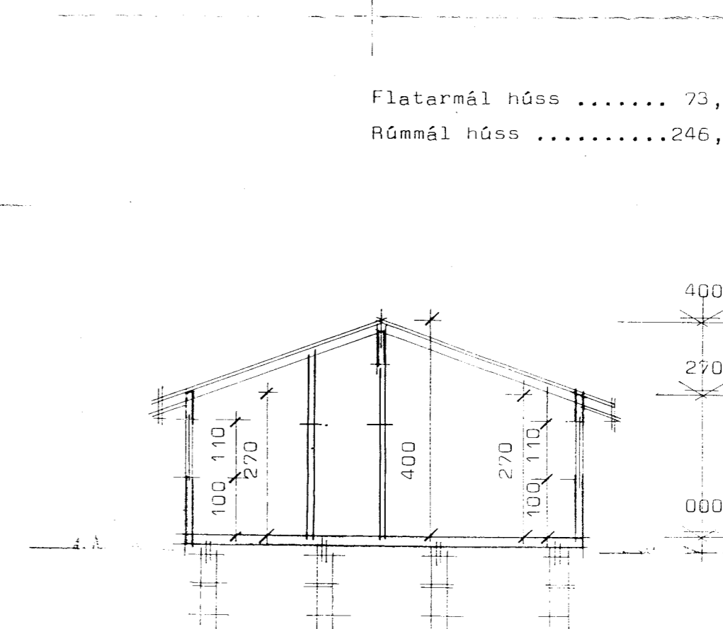
sneiðing
