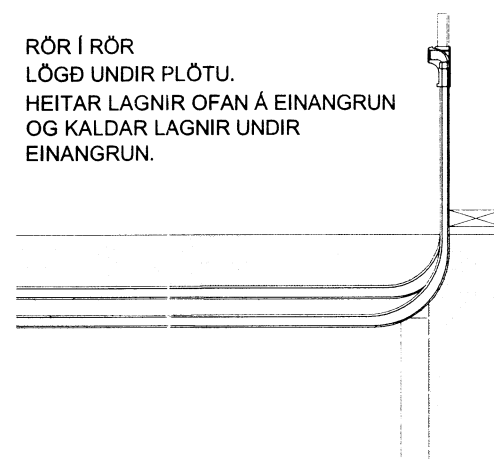
33 STAÐSETNING STÚTA VIÐ ÚTVEGG Mkv 1:20
