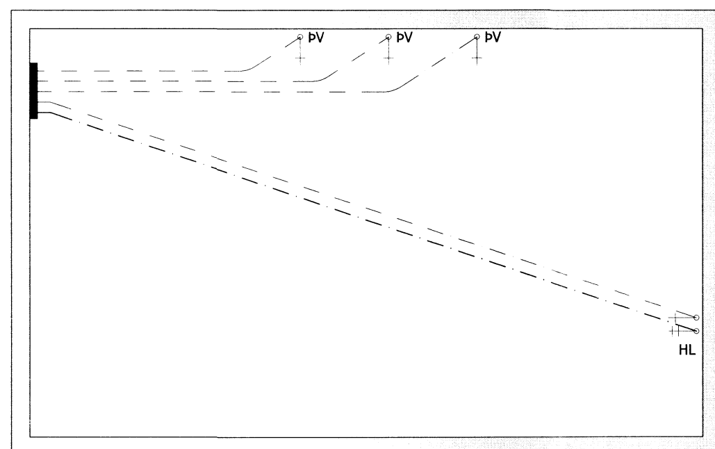
33 GRUNNMYND NEYSLUVATNSLAGNA Mkv 1:50
