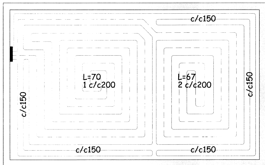
33 GRUNNMYND GÓLFHITALAGNA Mkv 1:50
