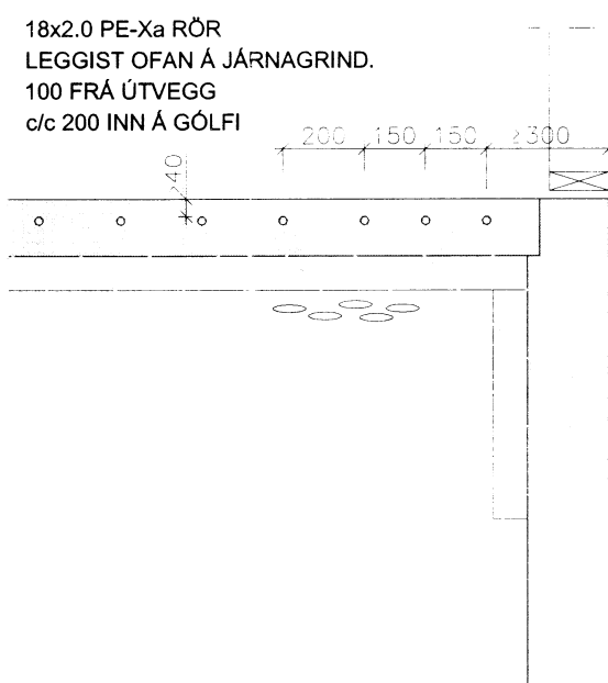
33 STAÐSETNING GÓLFGEISLA Í PLÖTU Mkv 1:20
