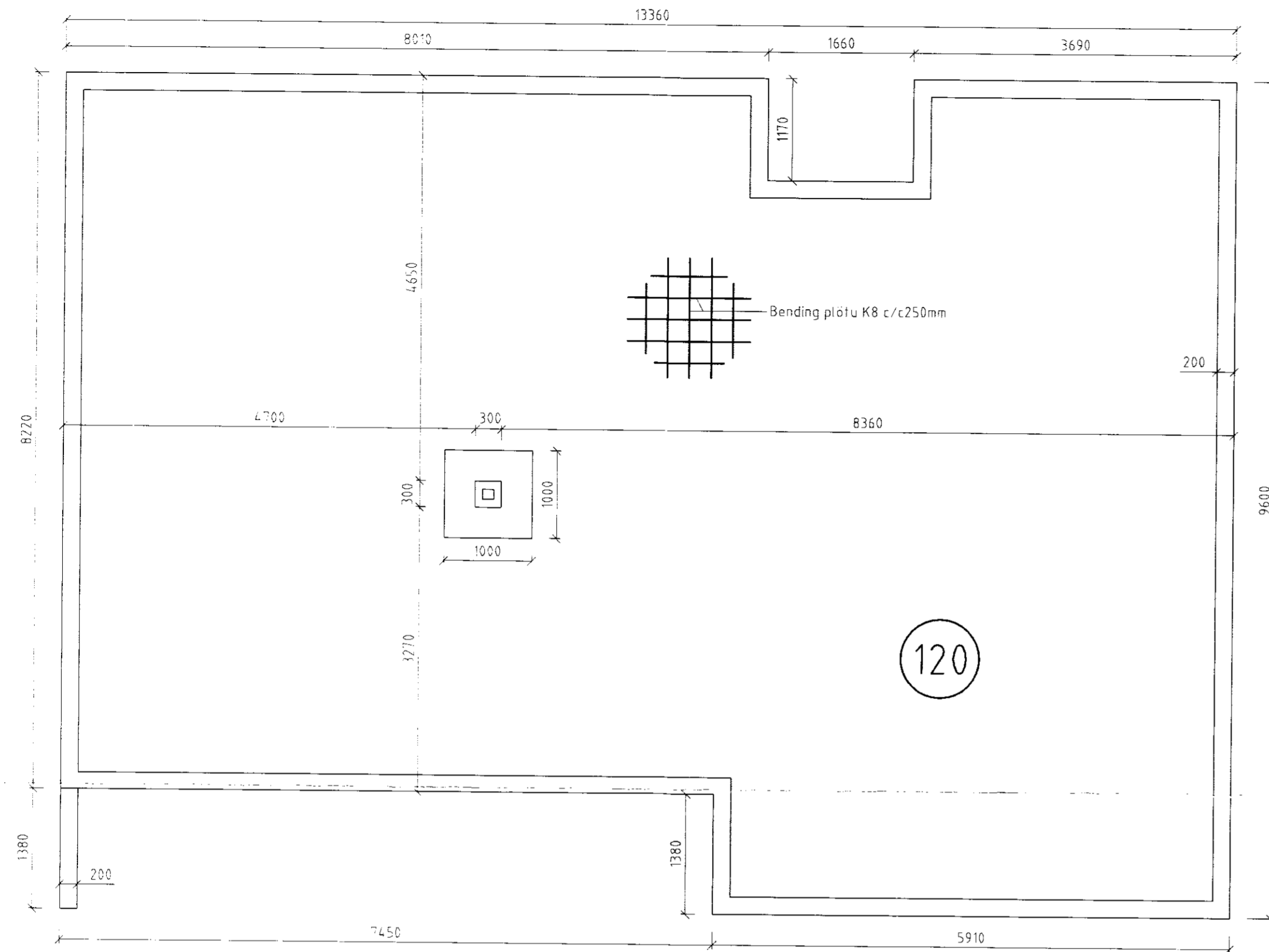
Grunnmynd söklla Mkv. 1:50
