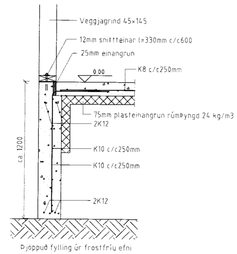
Snið 1 Mkv. 1:20
