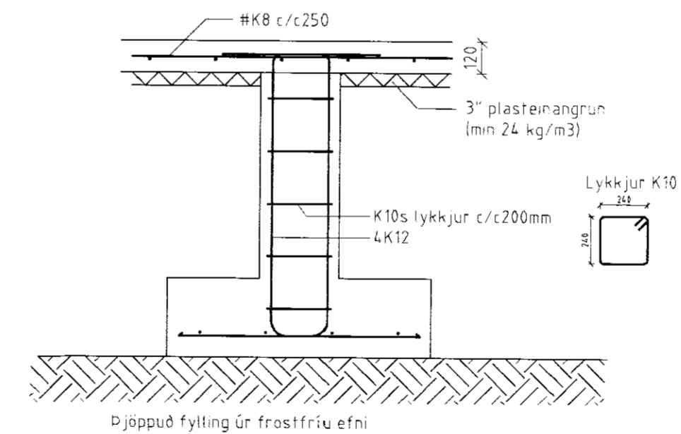
Sútur S1 - Mkv. 1:20
