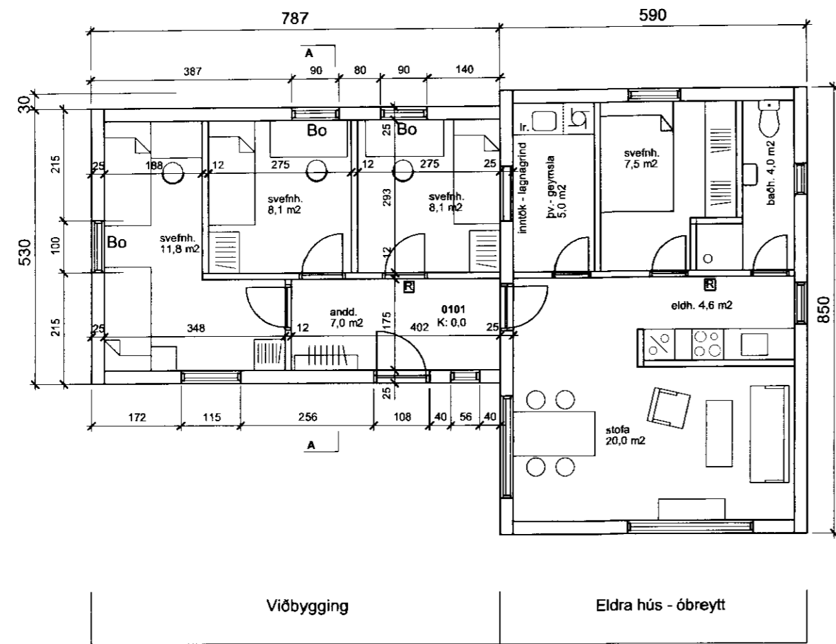
grunnmynd
