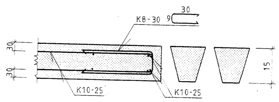
Snid P-P í plötukant. M=1:10
