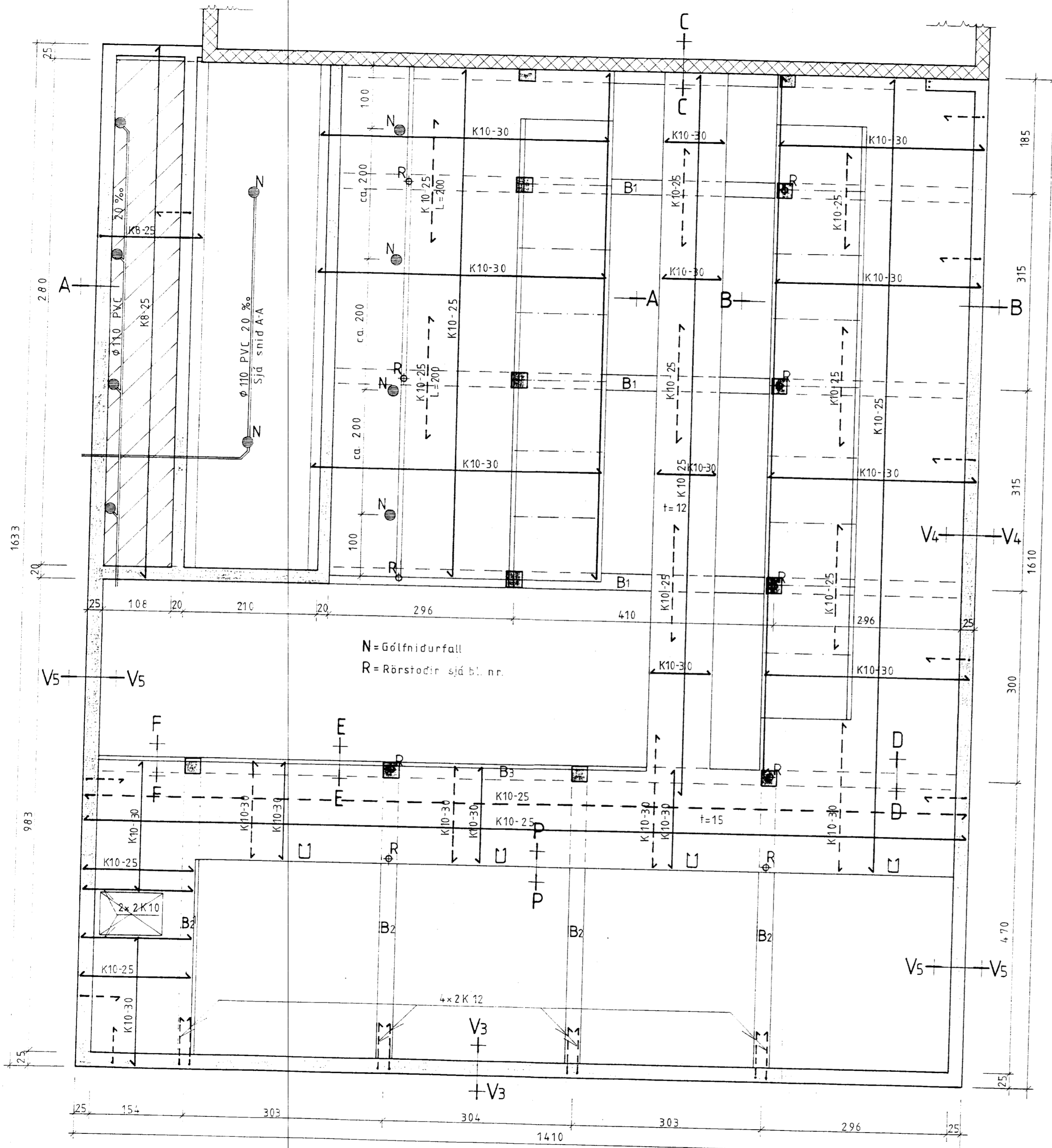
Gólf yfir haughúsi M=1:50
