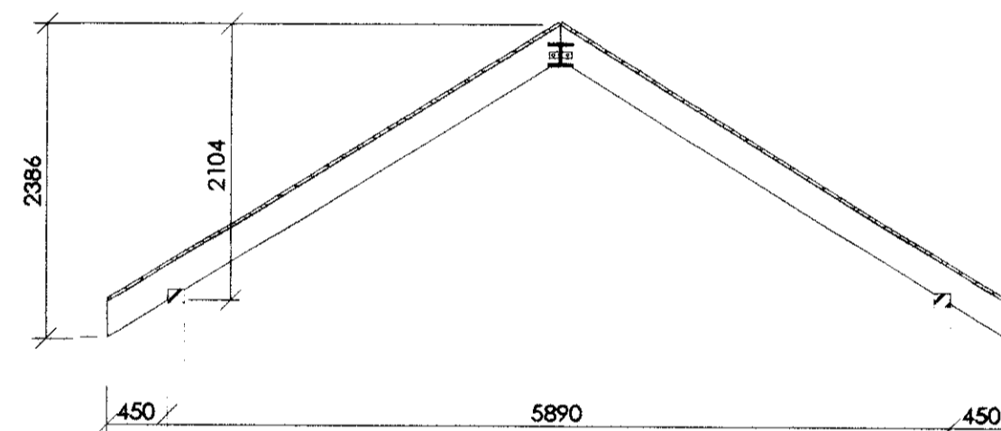
Snið B - B
