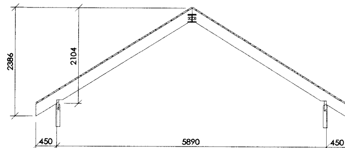
Snið C - C
