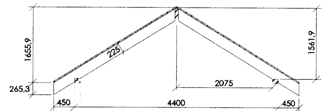
Snið A - A
