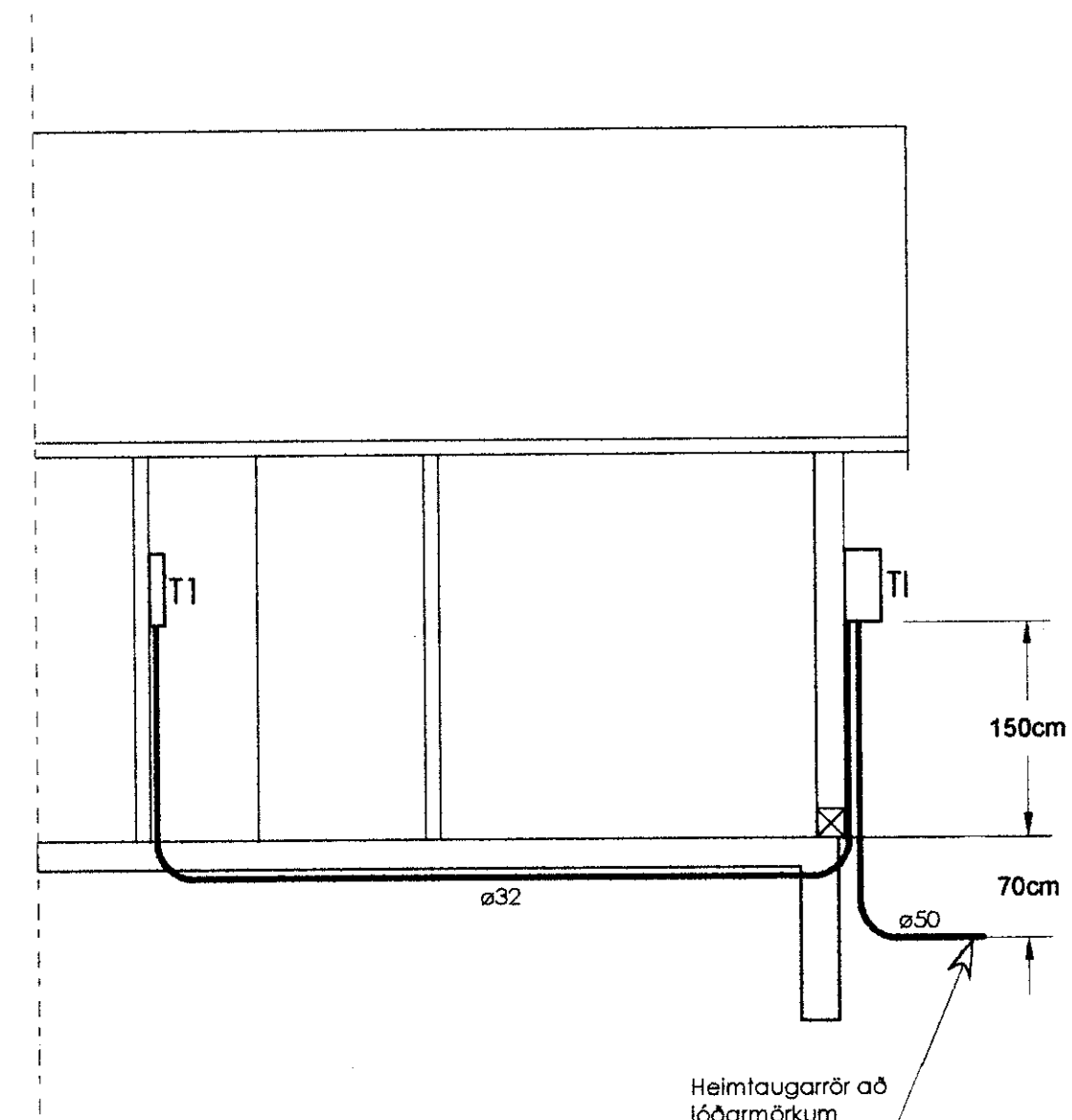
Snið 1:50
