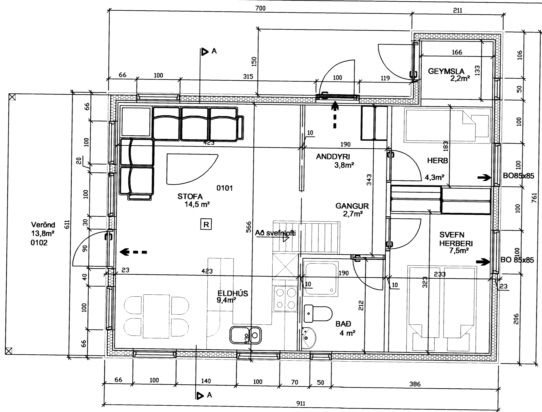
GRUNNMYND MKV. 1:50
