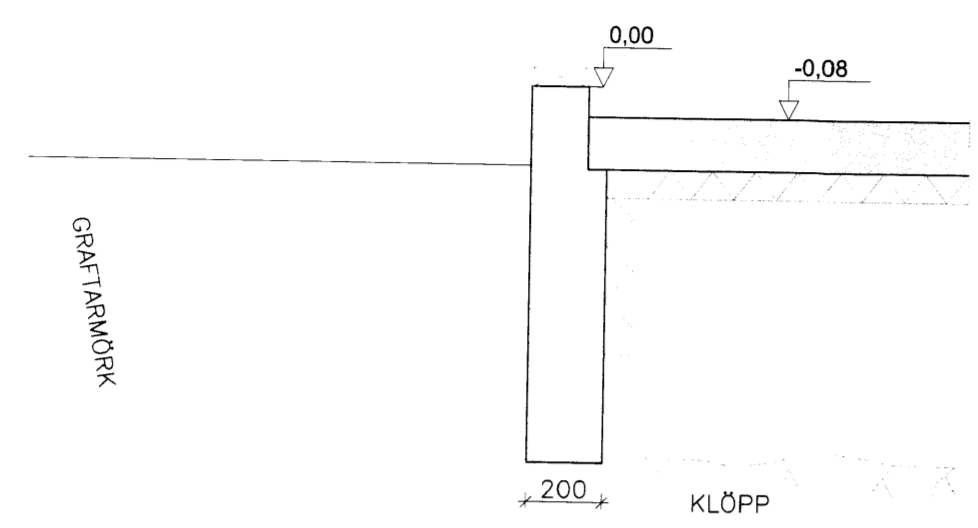
JARÐVINNUSNID
