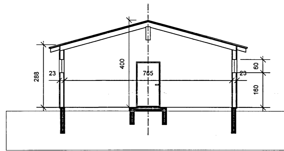
snið a-a
