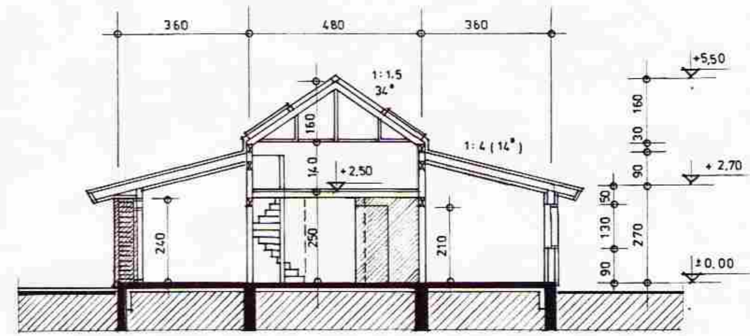
SNEIÐING A-A
