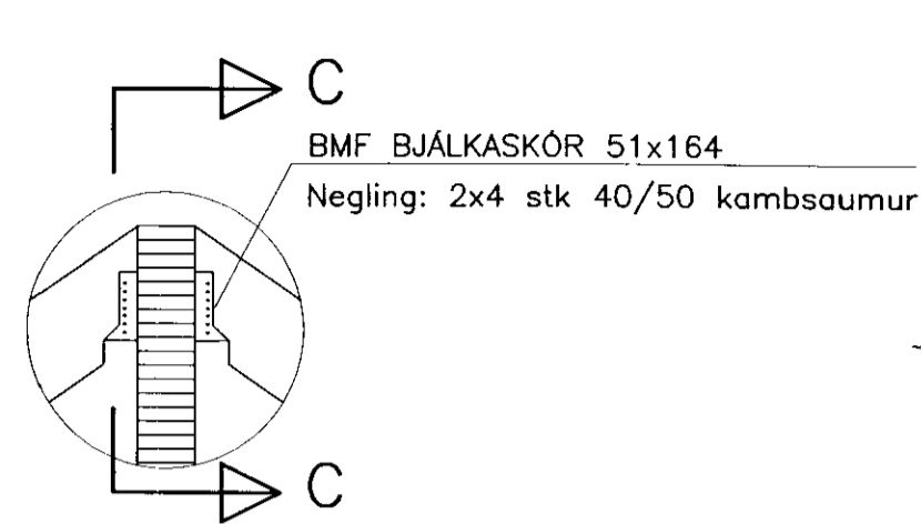
SÉRMYND 1 1:20
