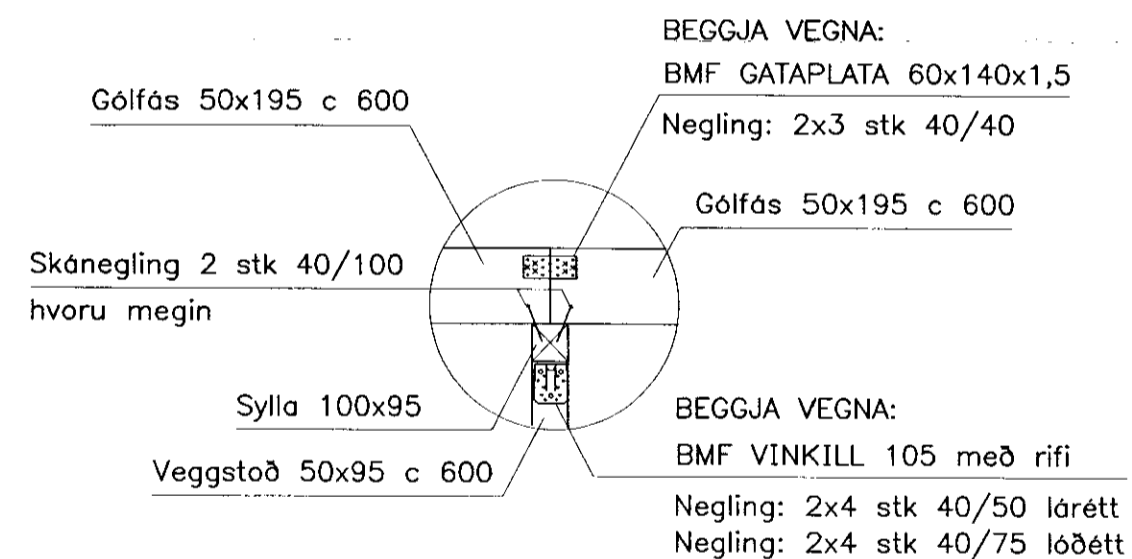
SÉRMYND 3 1:20
