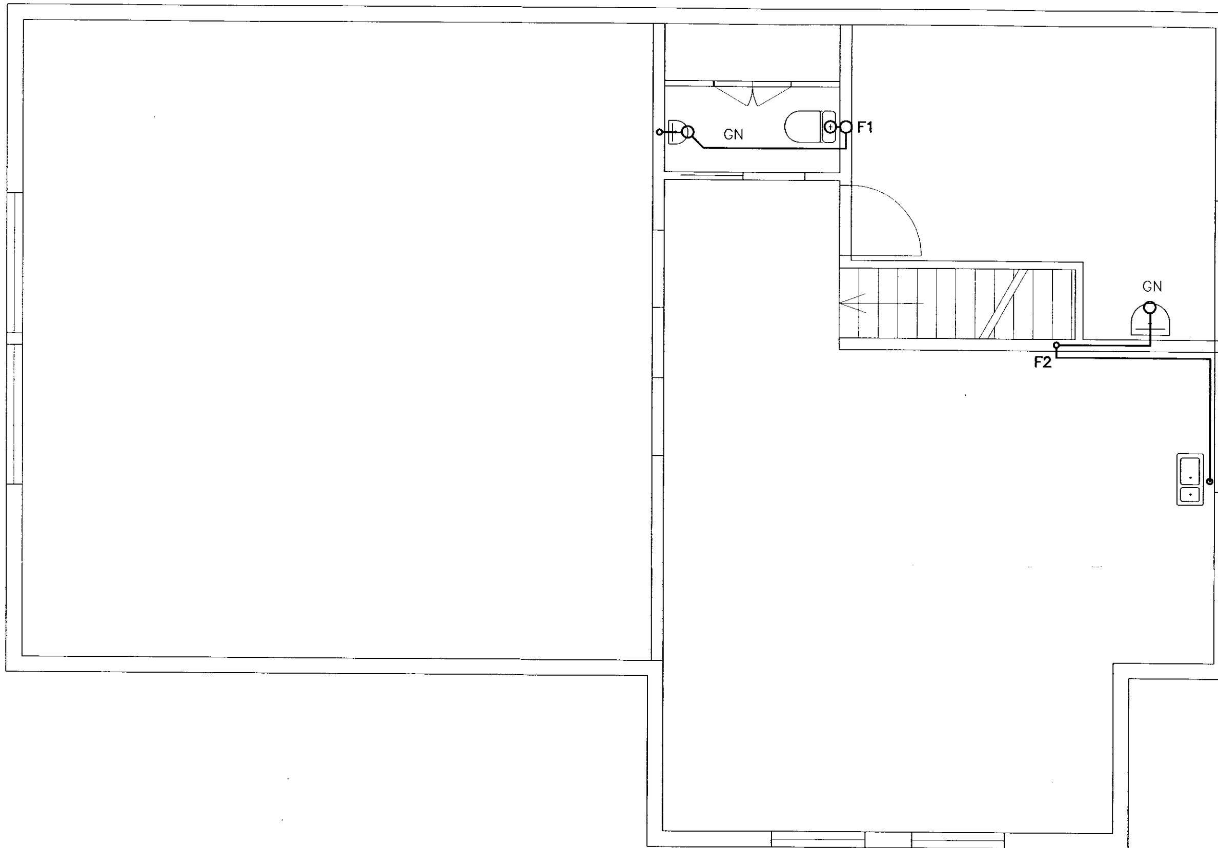
GRUNNMYND 1:50
