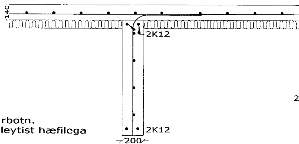
B - B
