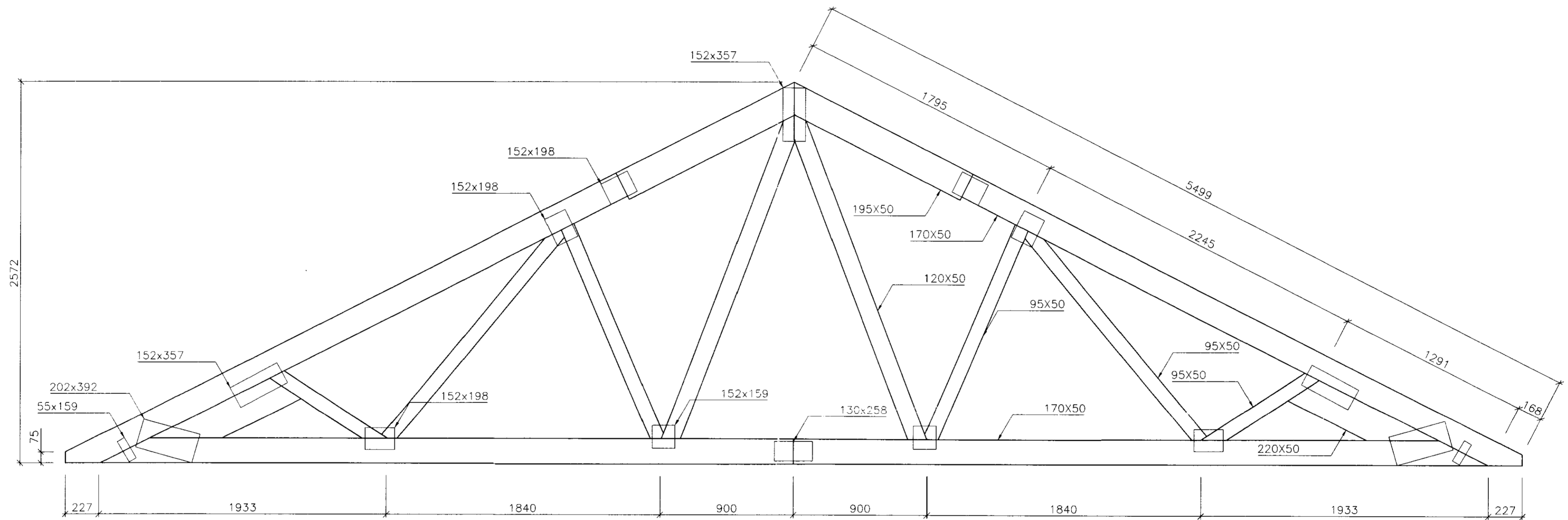
13 Snið S. 1:20
