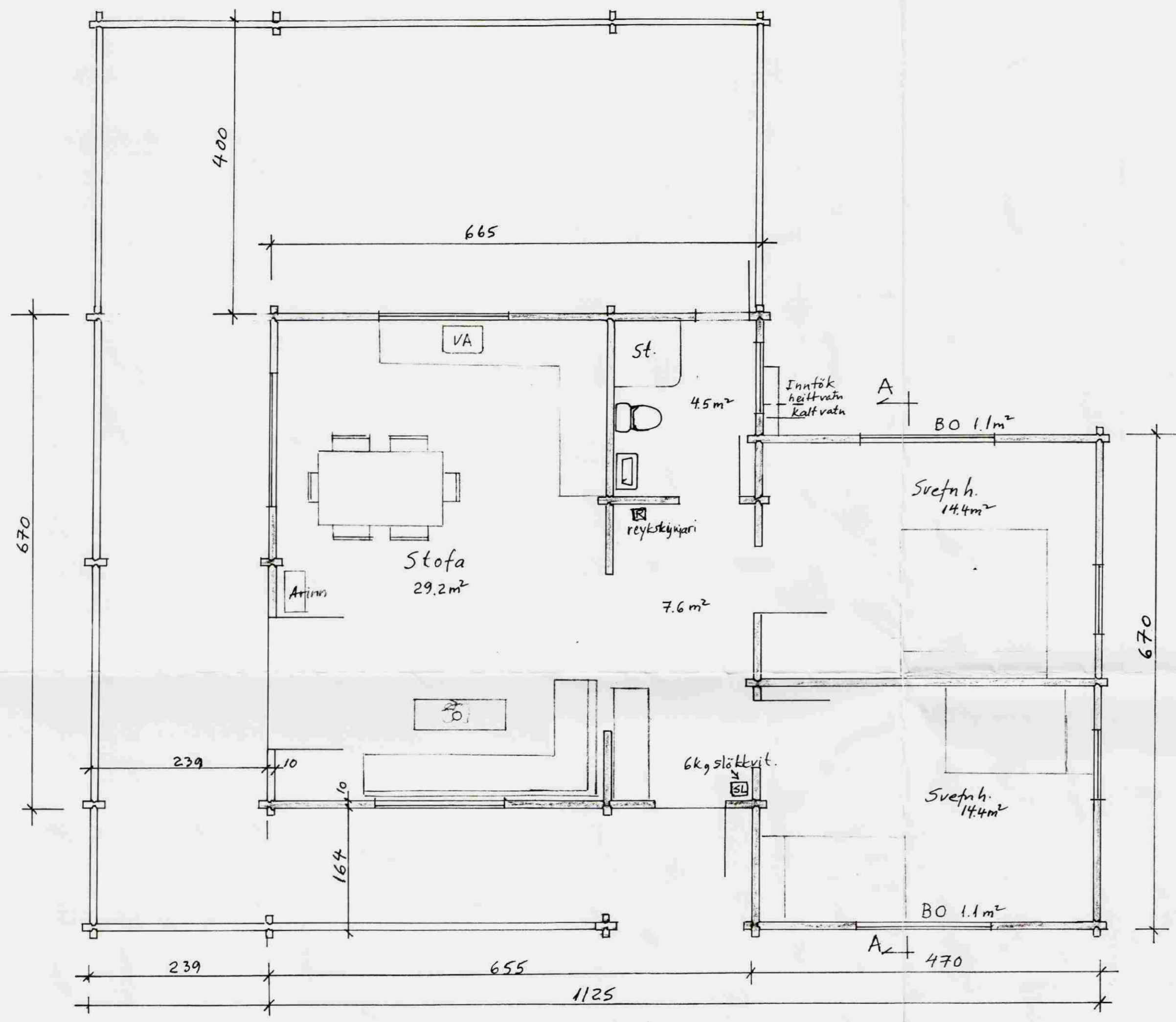
Grunnmynd; 1:50
