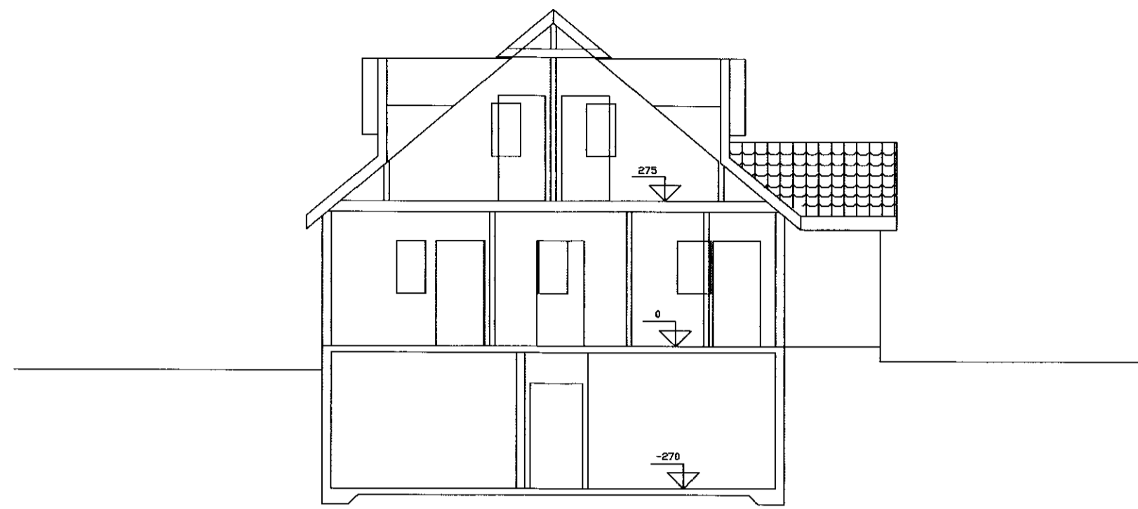
Snið A-A
