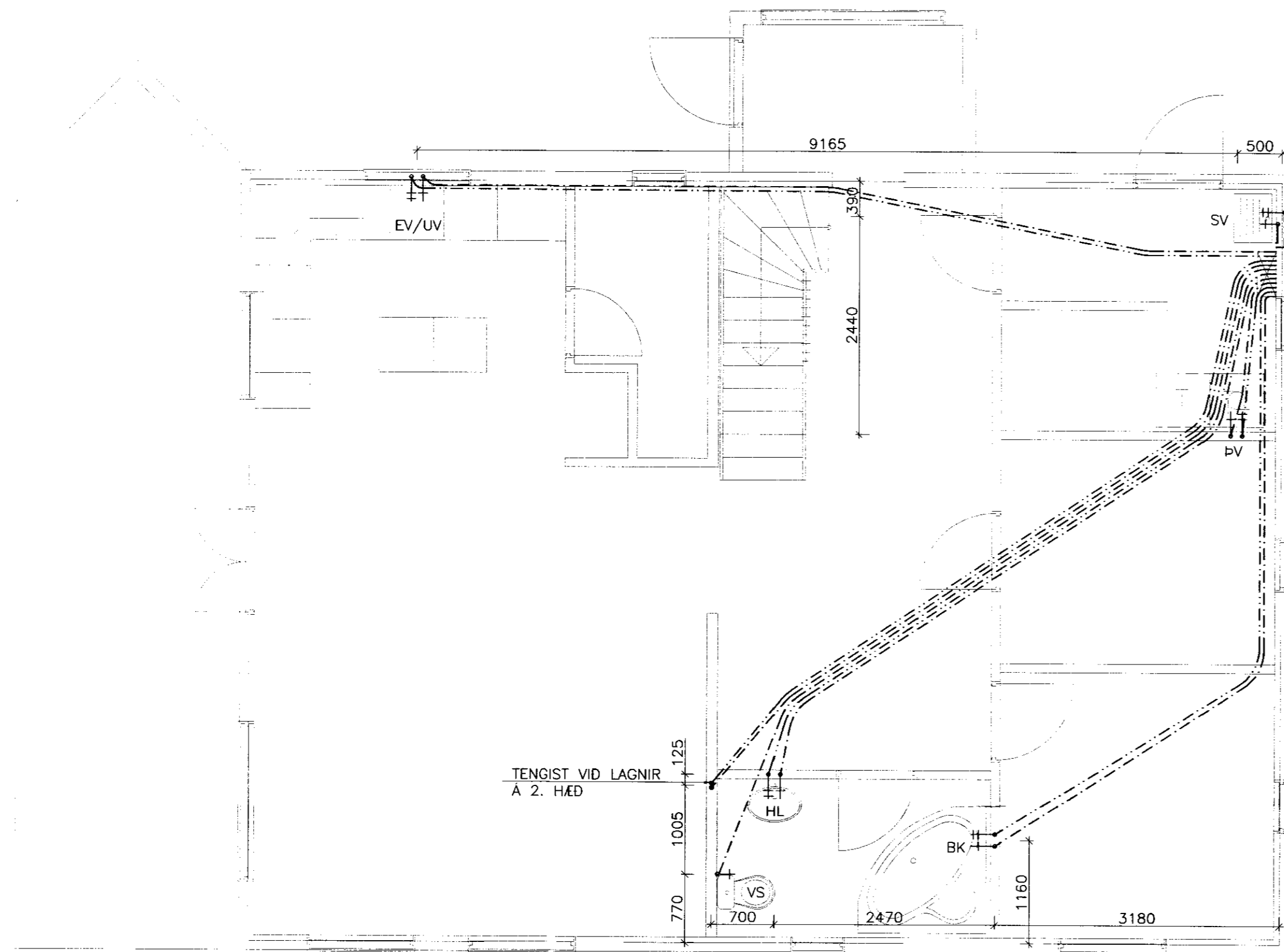
1. HÆÐ GRUNNMYND NEYSLUVATNSLAGNA 1:50
