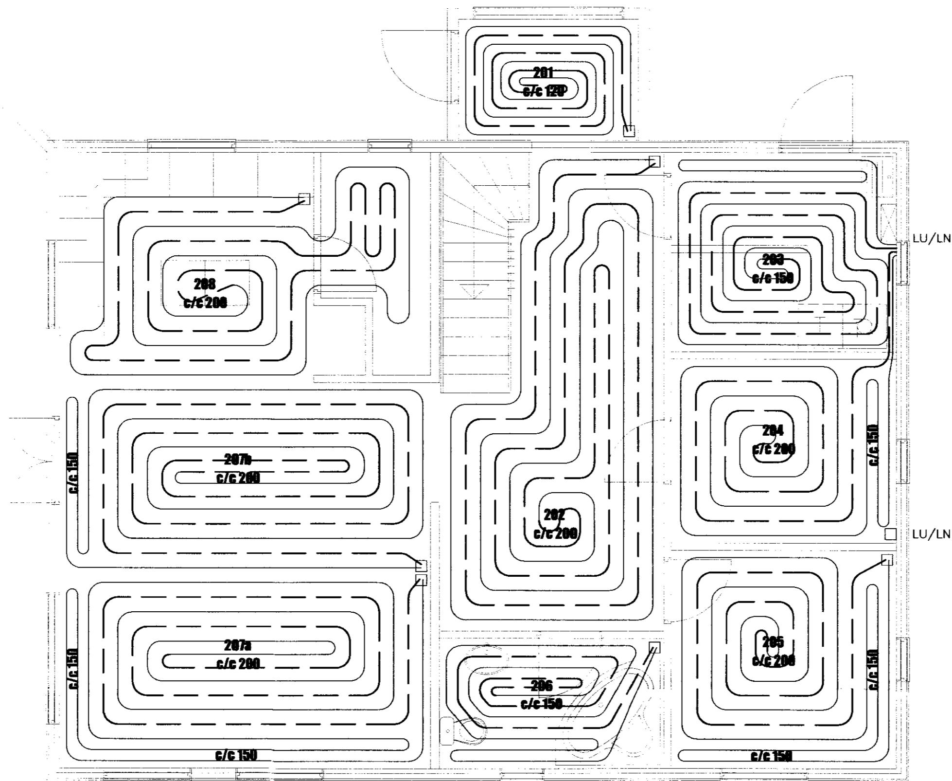
1. HÆÐ GRUNNMYND GÓLFGEISLALAGNA 1:50
