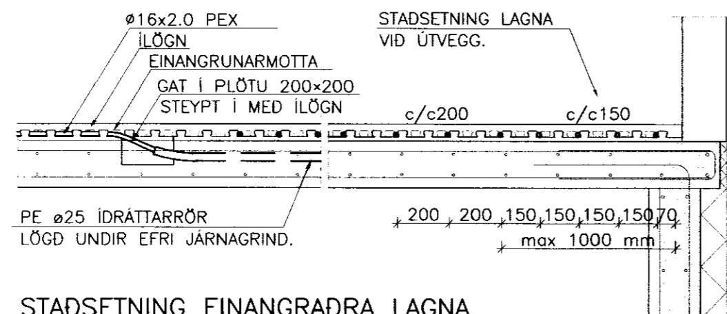
STADSETNING EINANGRADRA LAGNA Í GÓLFI Á 1. HÆÐ
