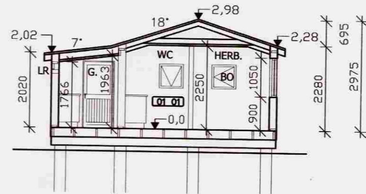
SNÍÐ A - A 1:100
