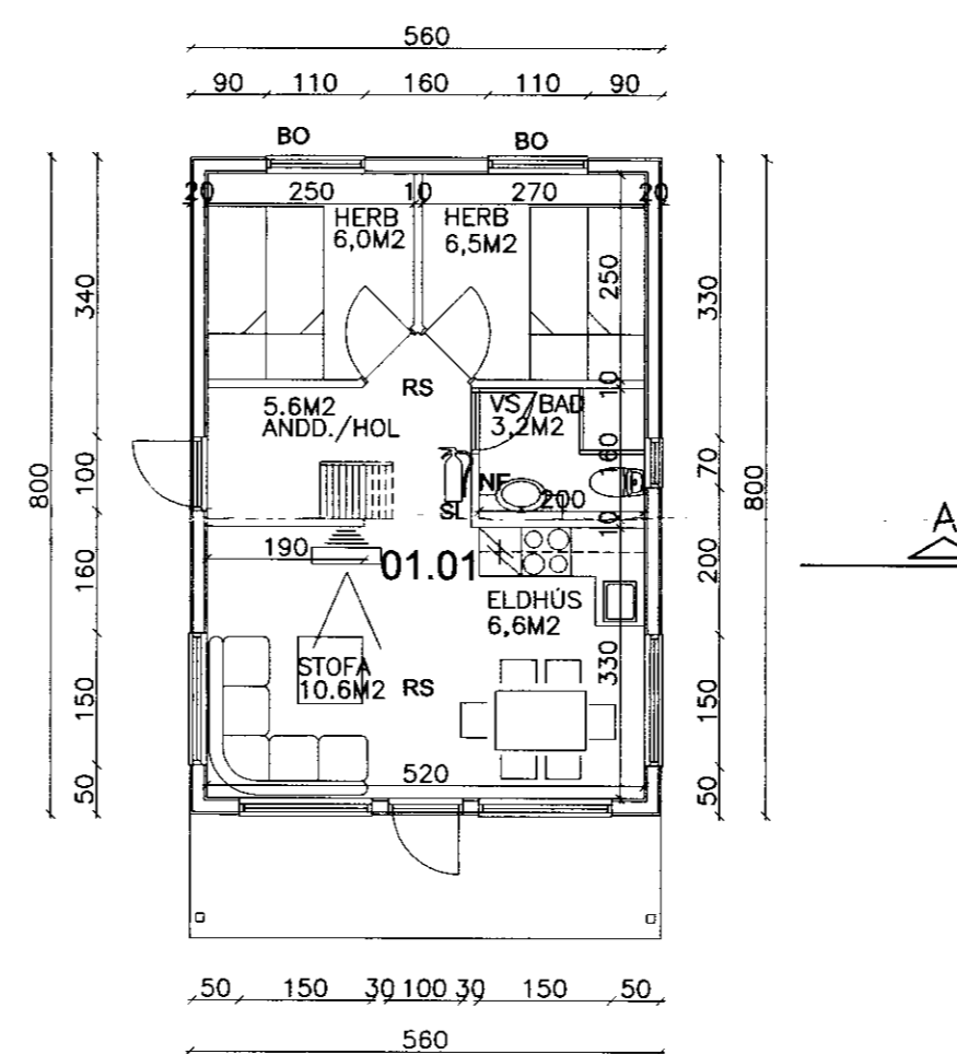
GRUNNMYND
