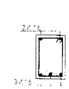
C-C M=1:20
