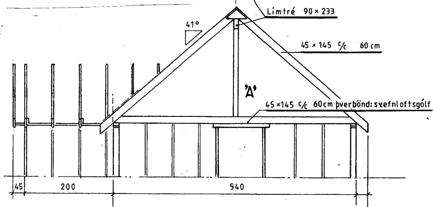
Snid A-A
