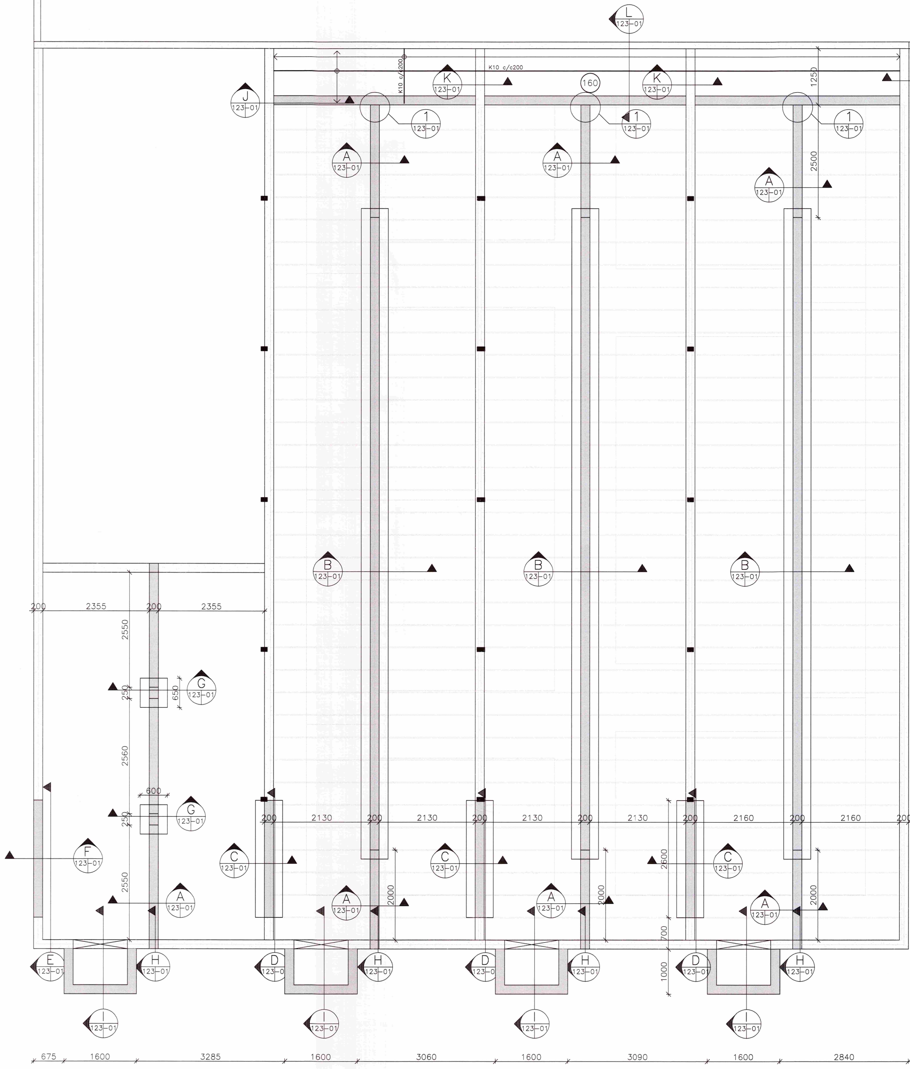
UNDIRSTÖÐUVEGGIR, GRUNNMYND 1:50
