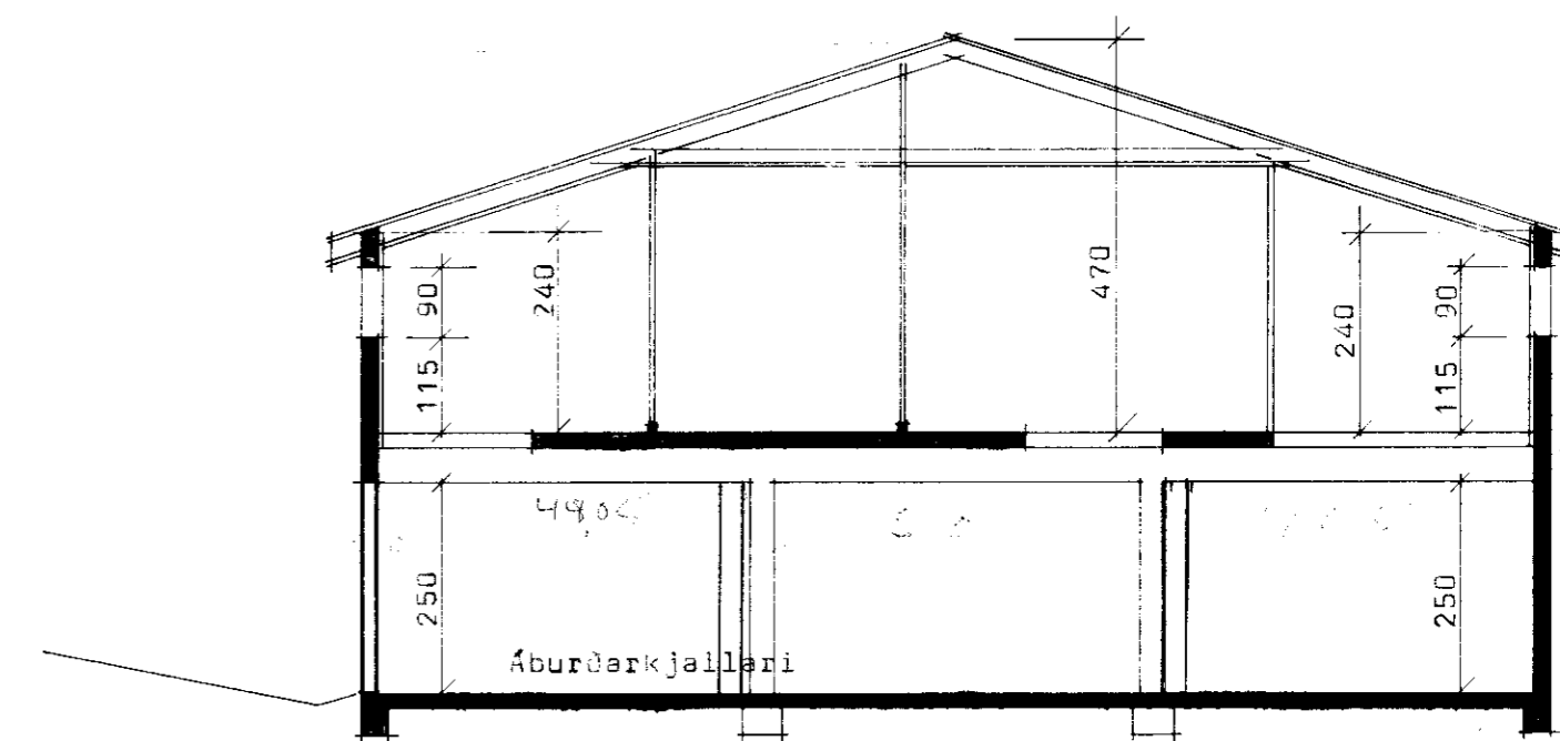
Skurður í fjósbyggingu
