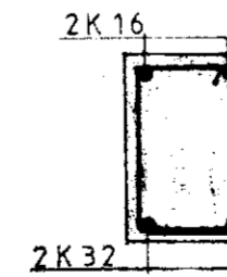
C-C M=1:20
