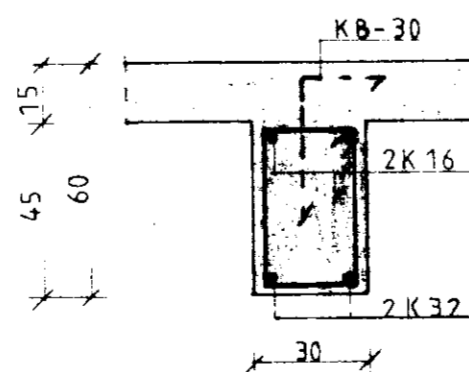
SNIÐ A-A M=1:20
