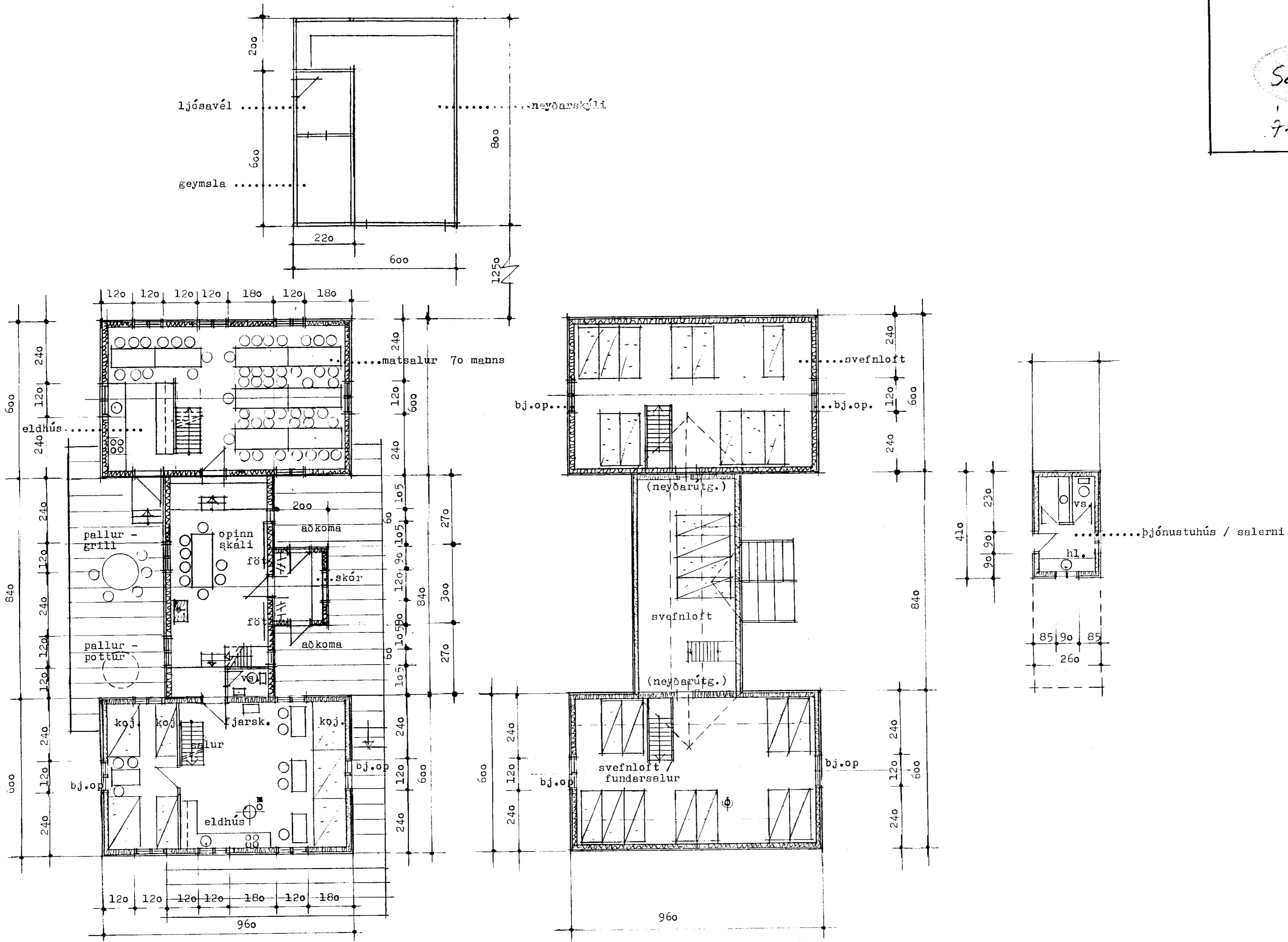
grunnmynd efri hæð 1:100
