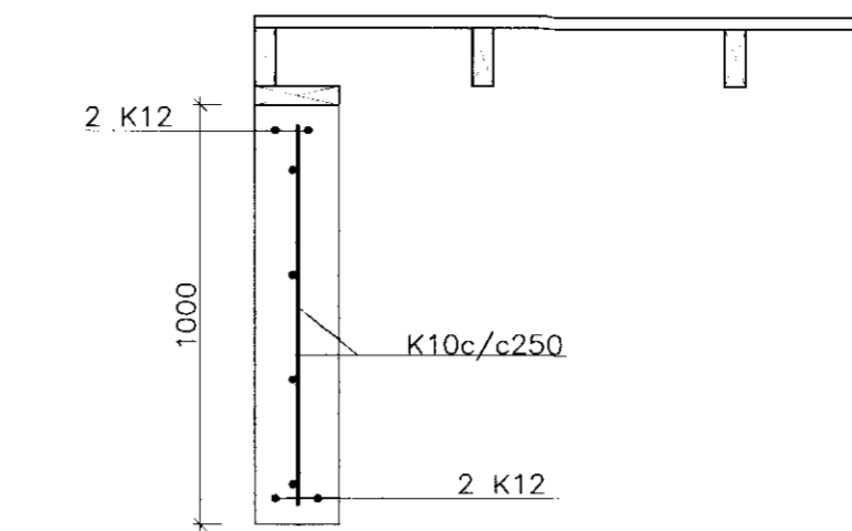
SNID Mkv: 1:20
