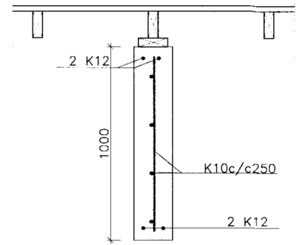
SNID Mkv: 1:20
