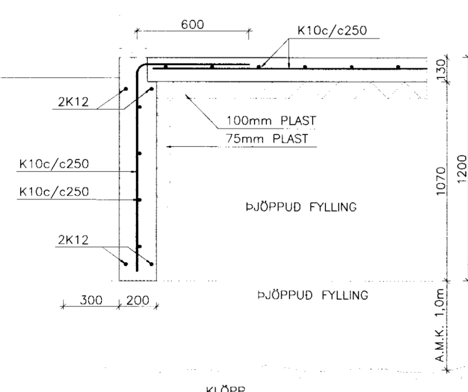
SNID Mkv: 1:20
