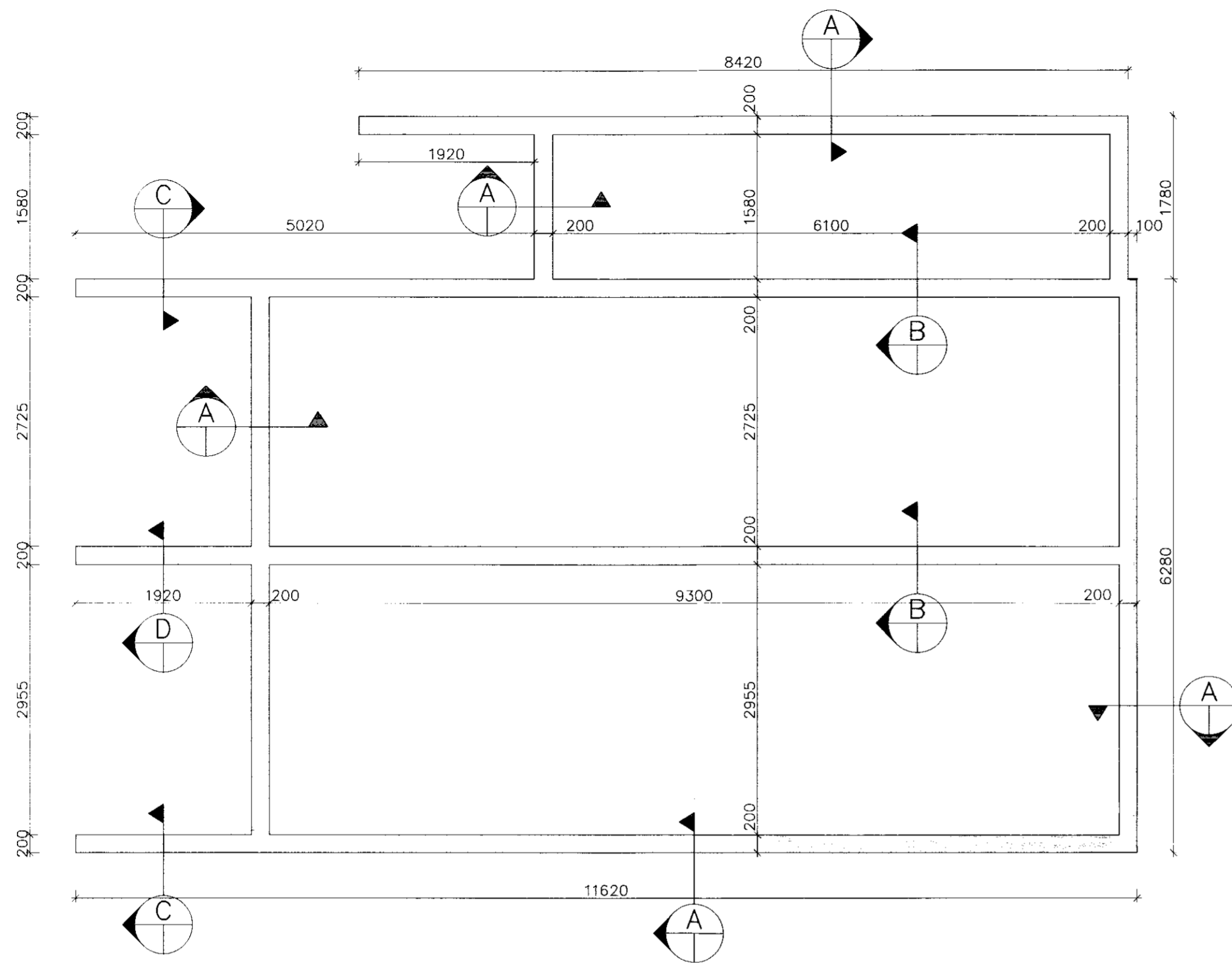
UNDIRSTÖÐUR, GRUNNMYND 1:50
