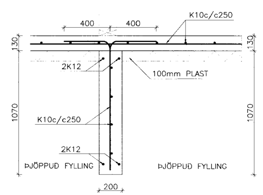
SNID Mkv: 1:20
