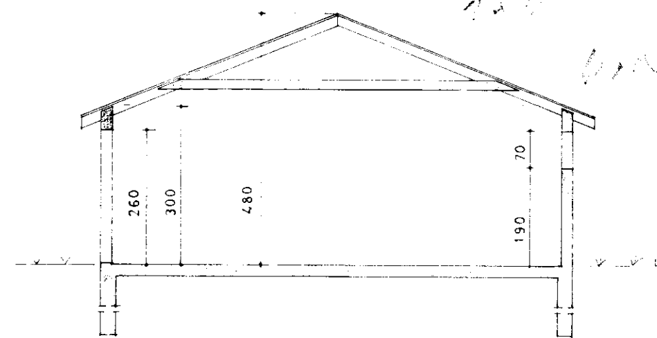
SNIÐ A-A
