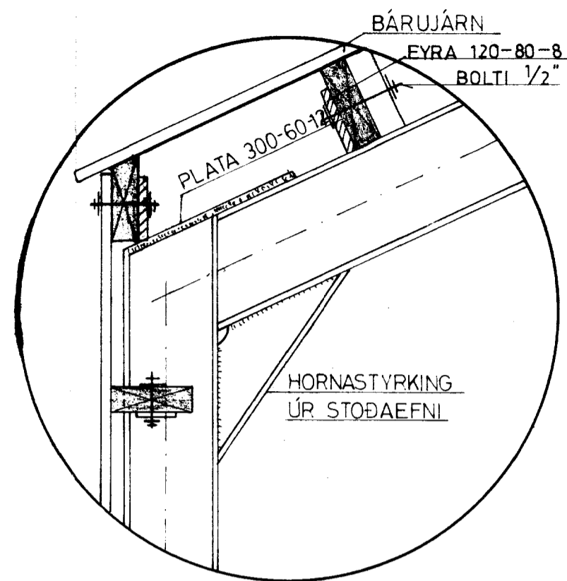
DEILI 1 M. 1:10
