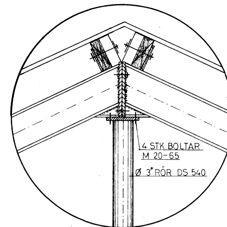
DEILI 3 M. 1:10
