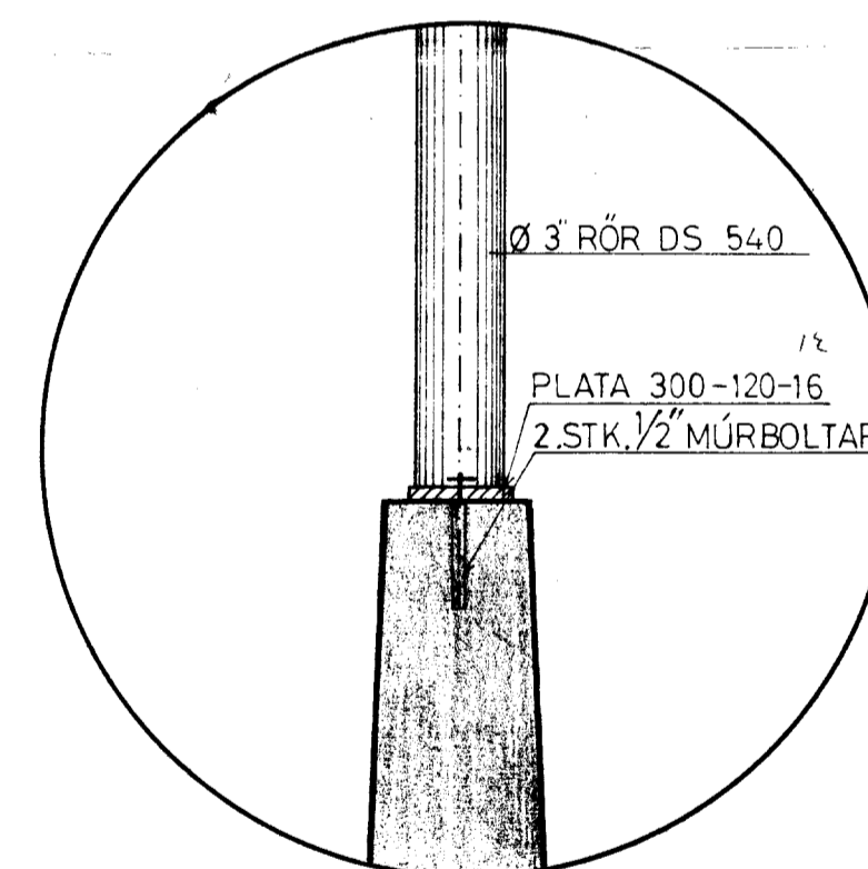
DEILI 4 M. 1:10
