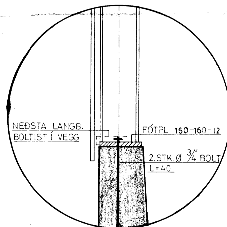
DEILI 2 M. 1:10
