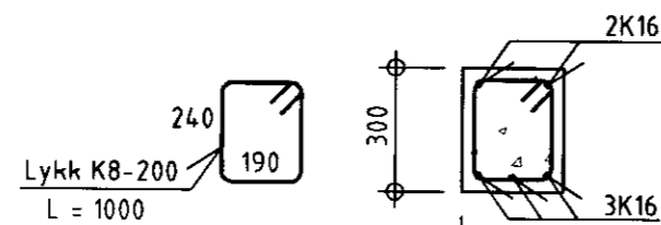
Snið B-B M = 1:20
