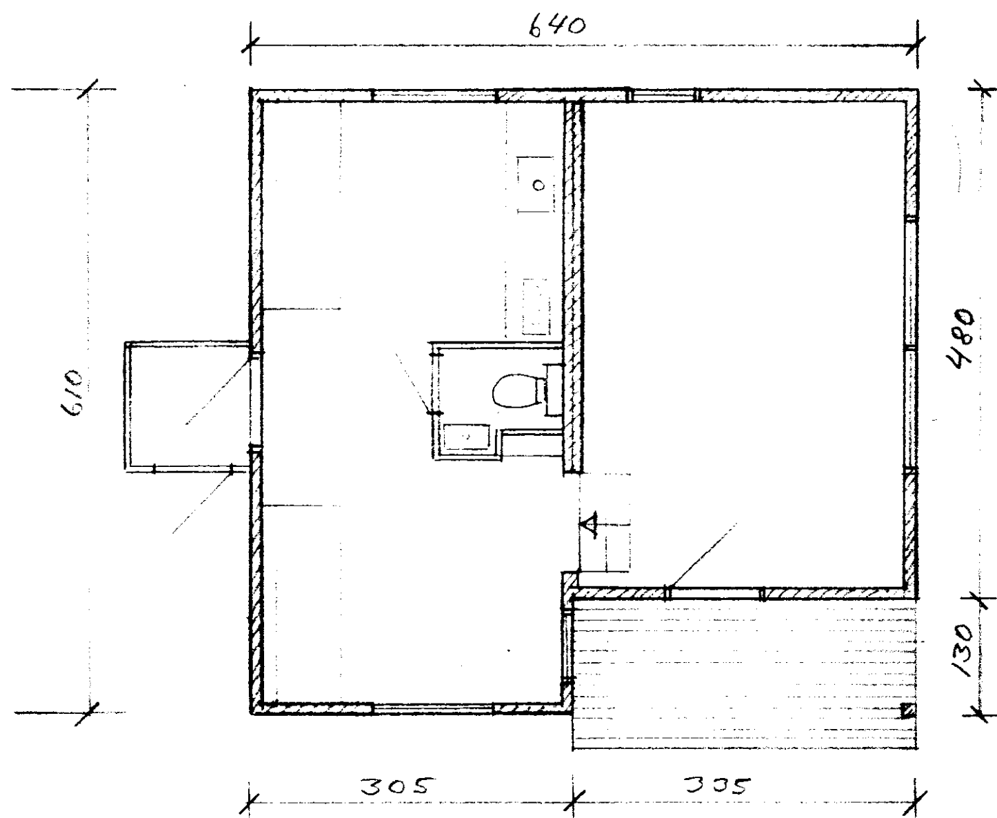
GRUNNMÝND 1:50
