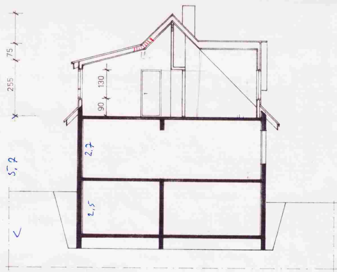
PVERSNID 1:100
