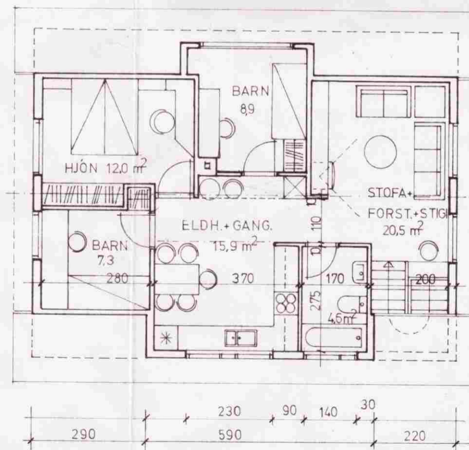
GRUNNMYND PAKHÆÐAR 1:100
