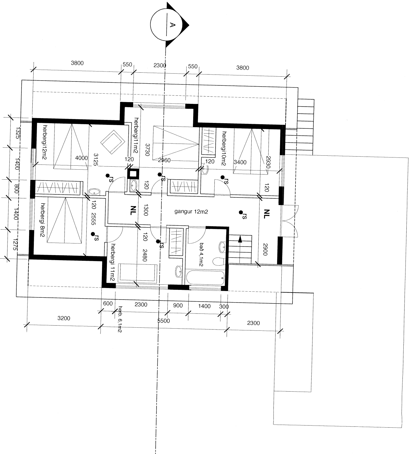
Grunnmynd rishæðar 1:100
