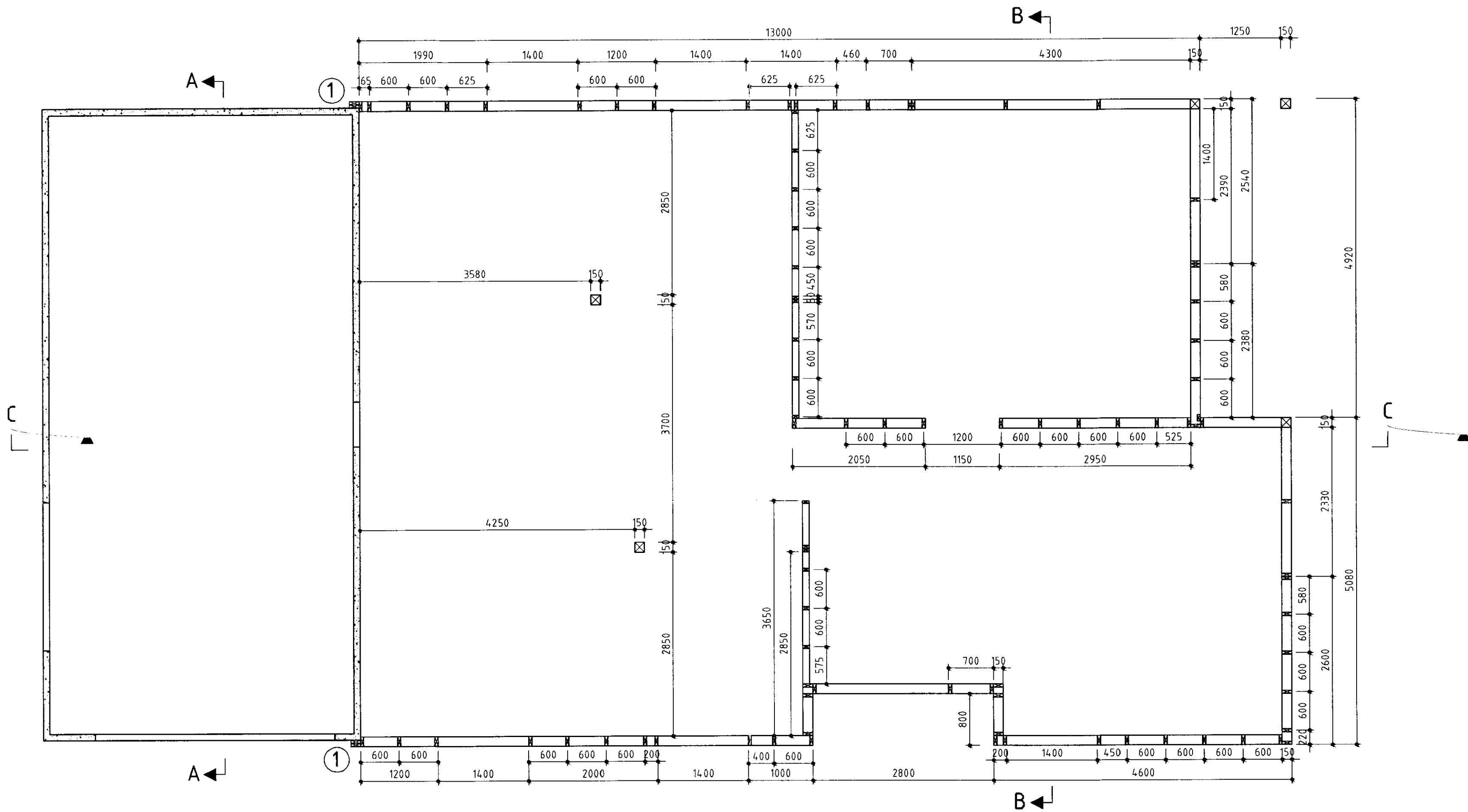
Timburgrind, grunnmynd Mkv. 1:50
